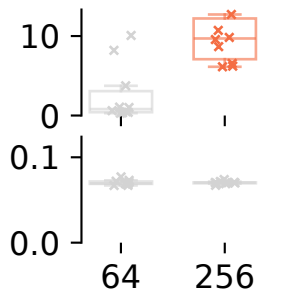
Straggling QoS (ms per update)
