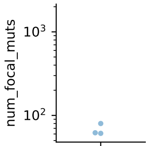
Sben1.1x Gneu
