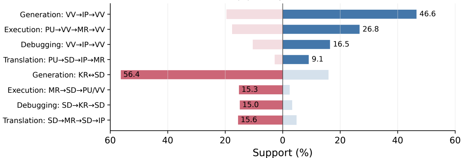
(b) R1-Qwen3-8B
