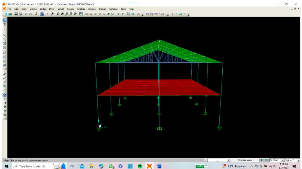
SAP2000 – BEBAN ANGIN KANAN
