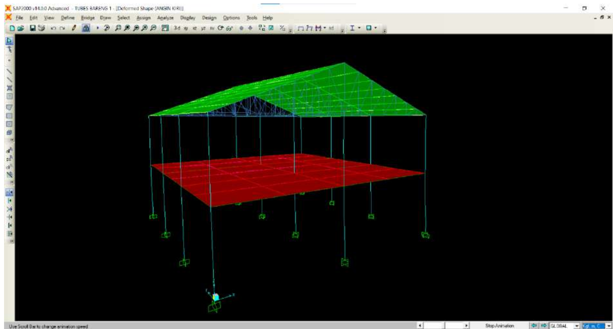
SAP2000 – BEBAN ANGIN KIRI
