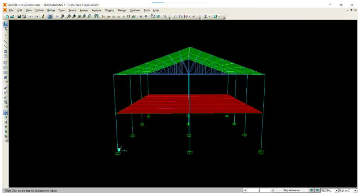
SAP2000 – BEBAN ATAP
