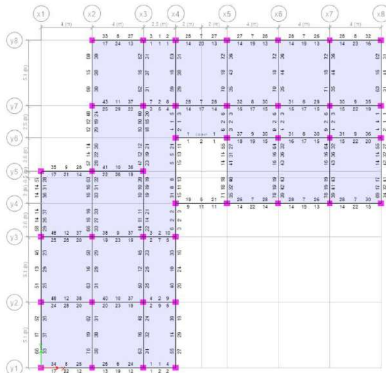
ETABS Lantai 2
