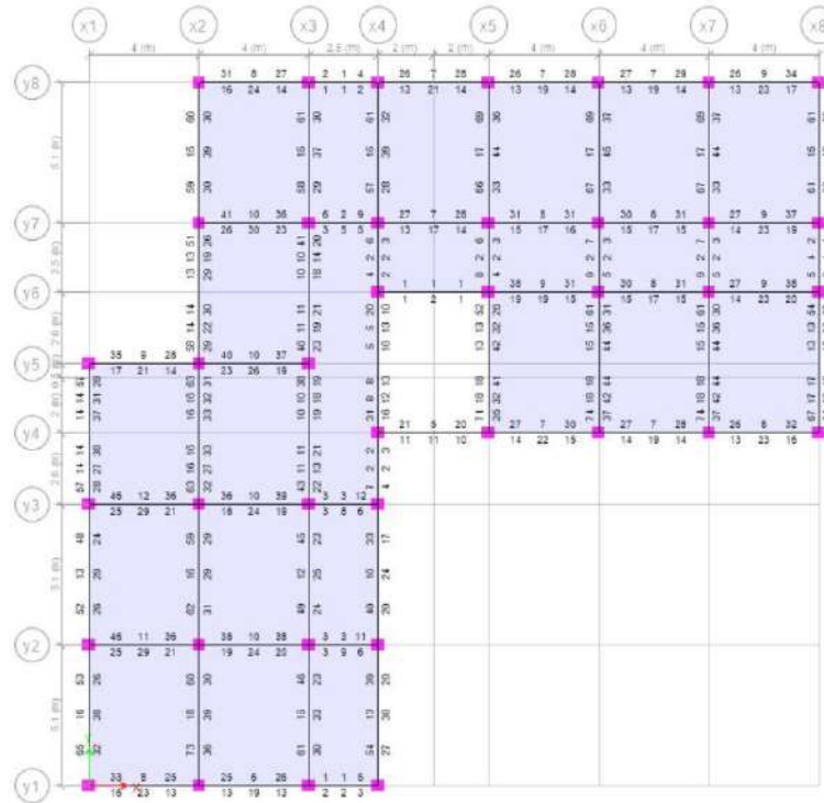
ETABS Lantai 3
