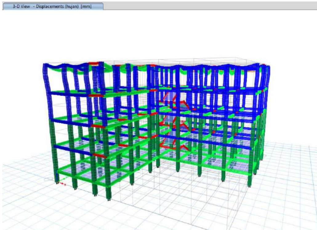
ETABS Beban Hujan
