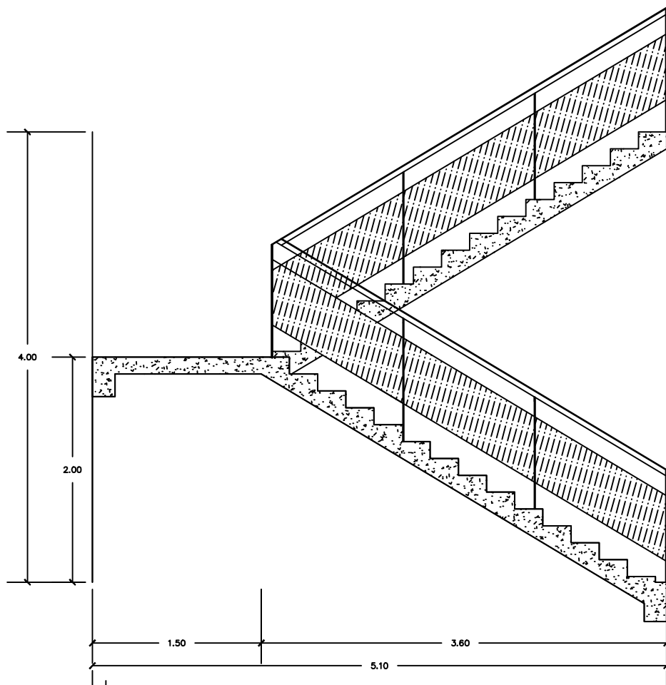
Model Tangga SKALA 1 : 100
