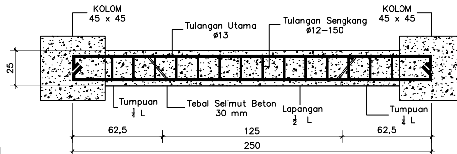
Potongan balok induk koridor Arah Y SKALA 1 : 100
