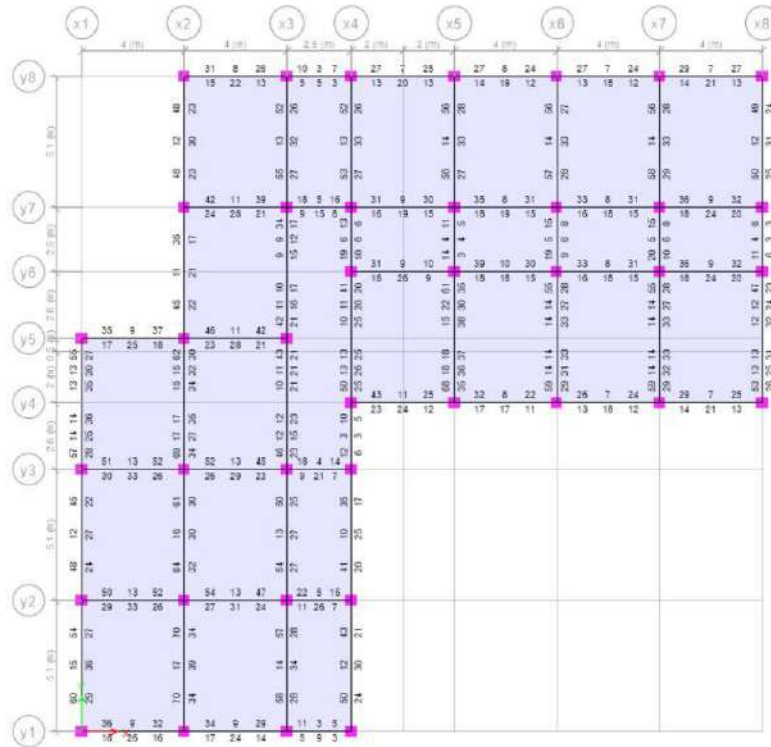
ETABS Lantai 1
