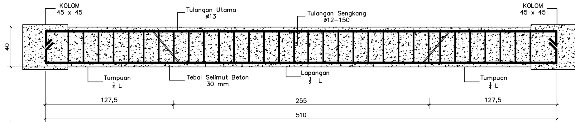
Potongan balok induk Arah Y SKALA 1 : 100
