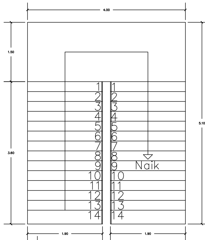
denah Tangga SKALA 1 : 100
