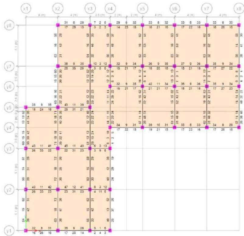
ETABS Atap
