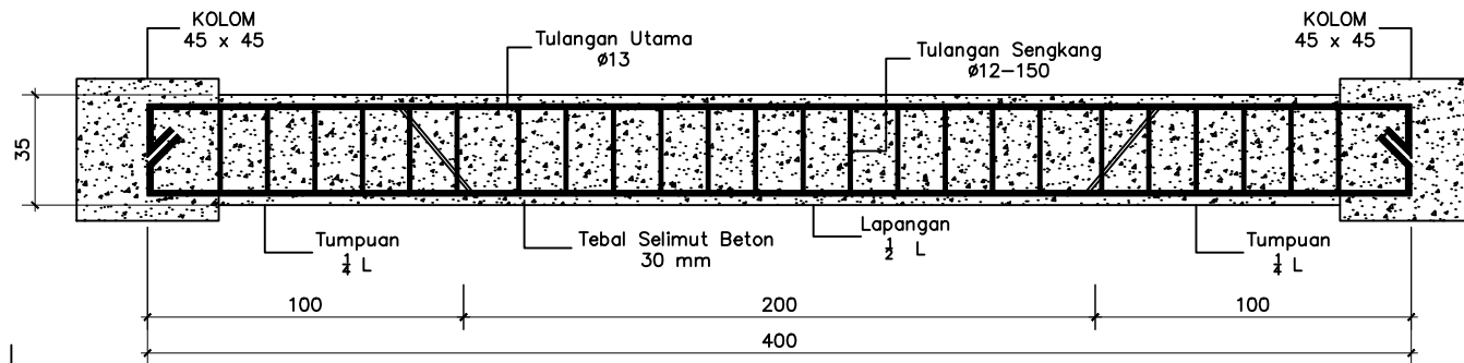
Potongan balok induk Koridor Arah X SKALA 1 : 100
