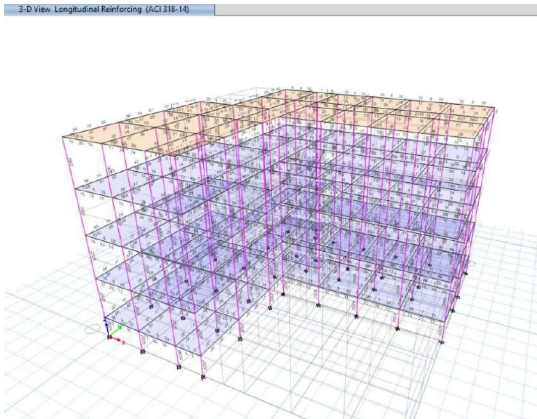
Etabs Tampak 3 dimensi
