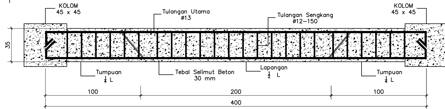
Potongan balok induk Arah X SKALA 1 : 100
