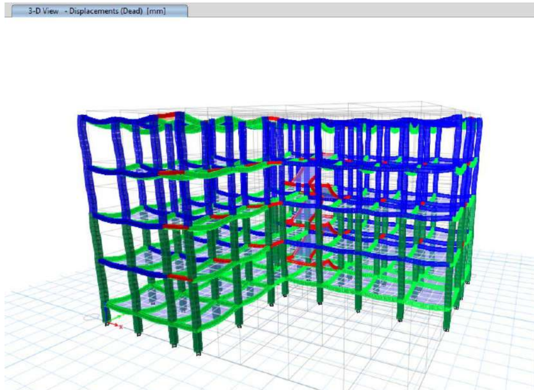
ETABS Beban Mati
