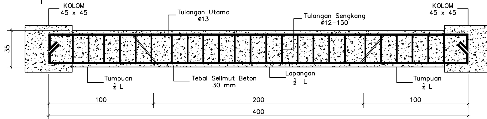
Potongan Sloof X SKALA 1 : 100
