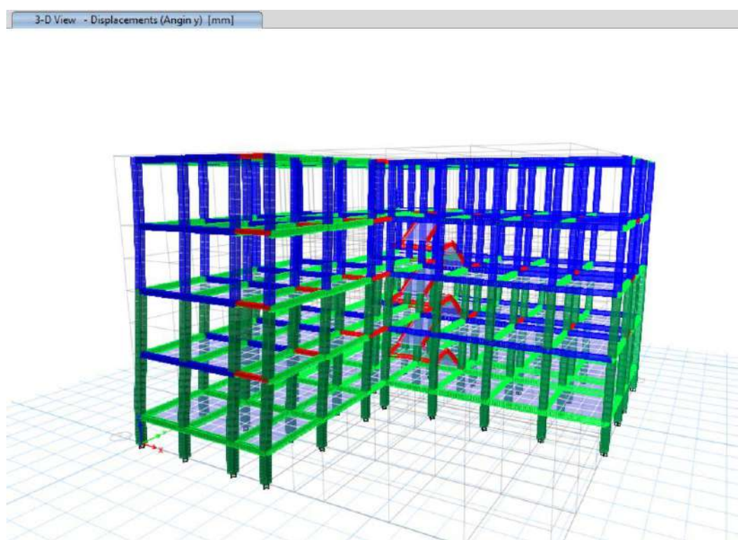
ETABS Beban Angin Y
