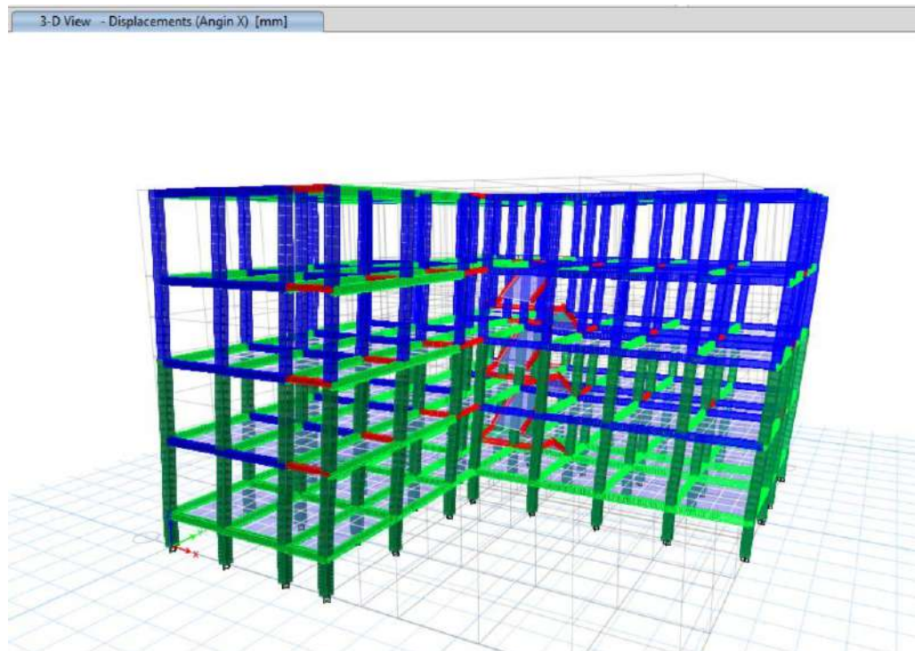
ETABS Beban angin X
