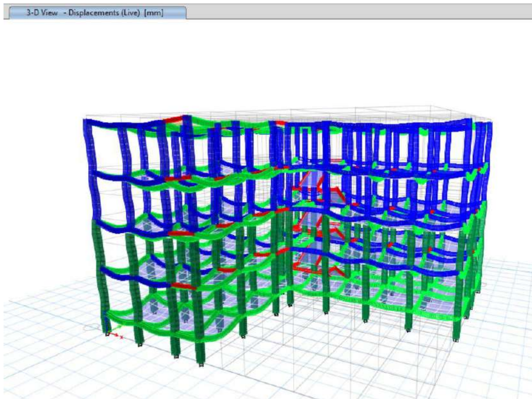
ETABS Beban Hidup
