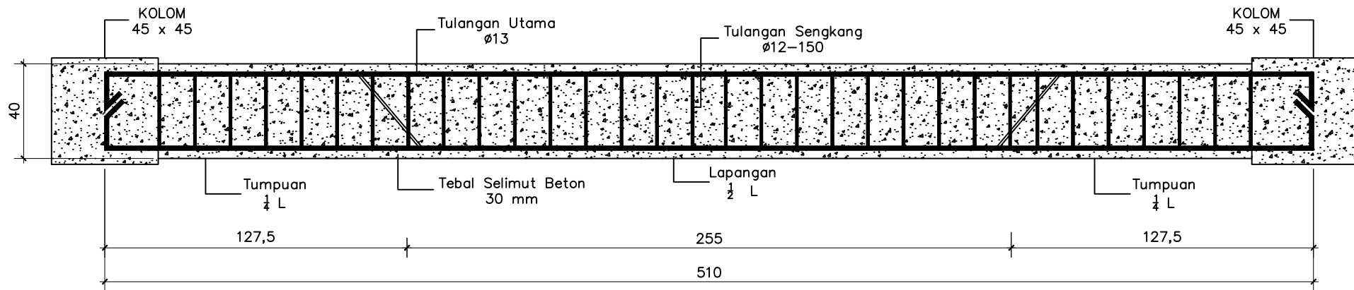
Potongan Sloof Y SKALA 1 : 100
