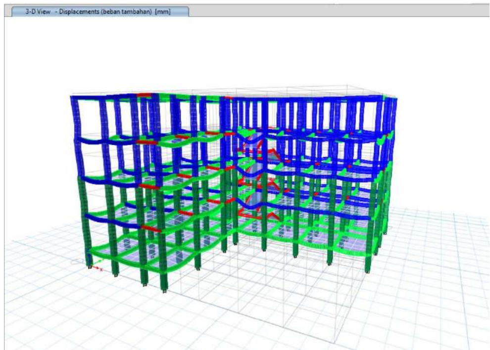
ETABS Beban Tambahan
