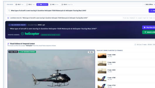
(d) VQA: Grounded Answer &amp; Evidence Timeline (Helicopter)
