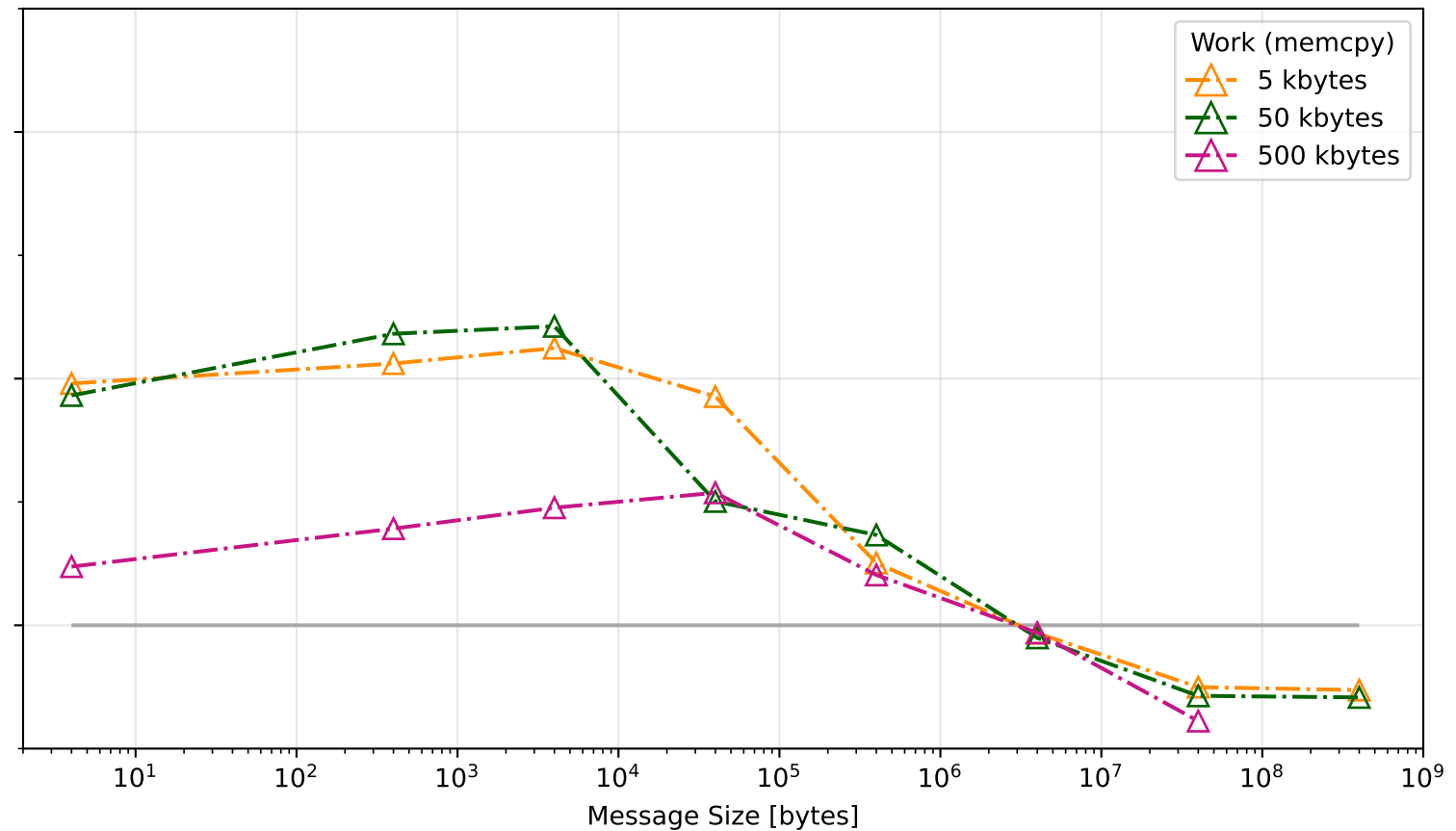
SNG: Intel Xeon(R) Gold 6148 48 Cores (2 Nodes, 1 MPI proc per Socket, 23 threads per MPI proc)
