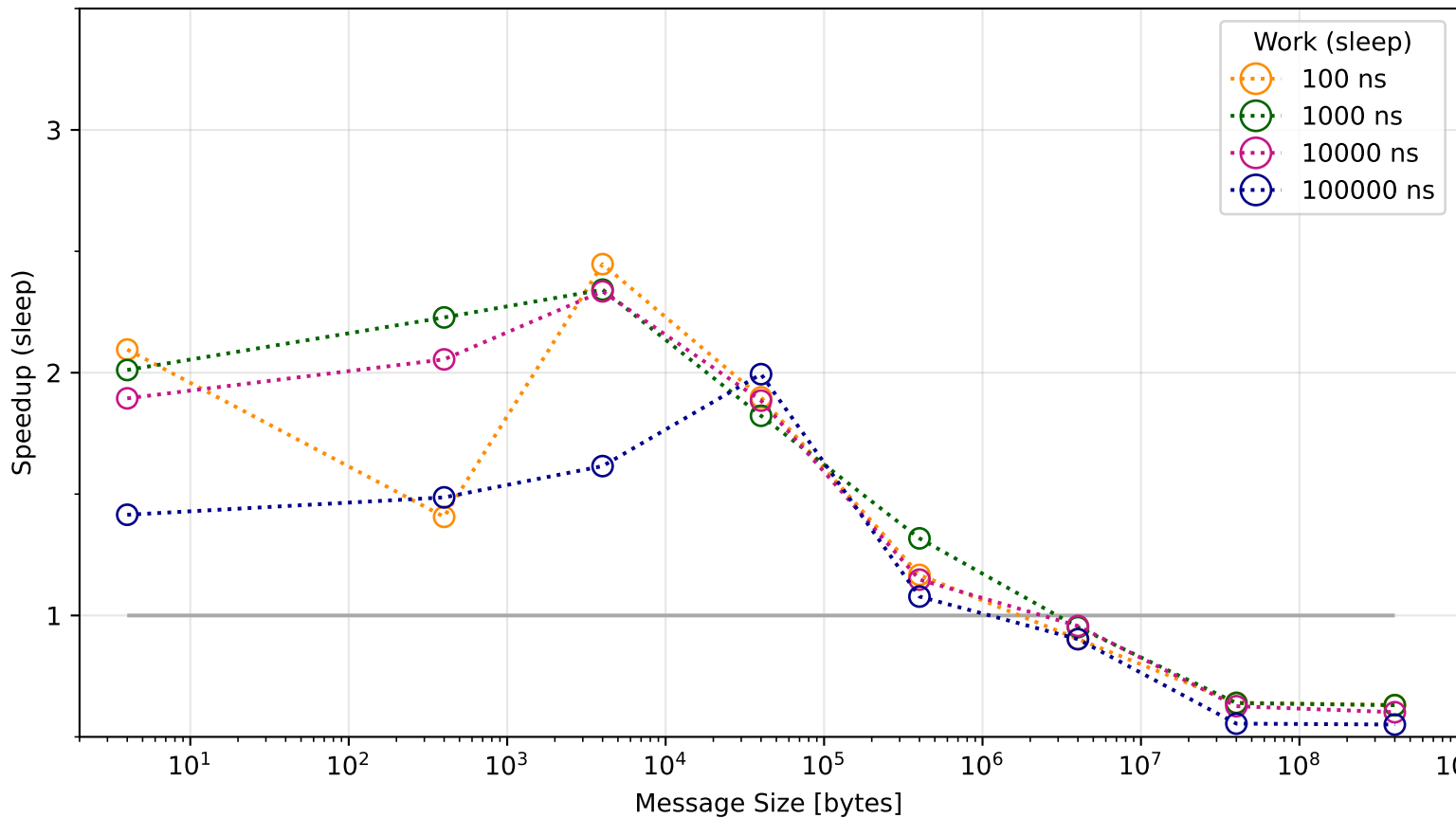
SNG: Intel Xeon(R) Gold 6148 48 Cores (2 Nodes, 1 MPI proc per Socket, 23 threads per MPI proc)
