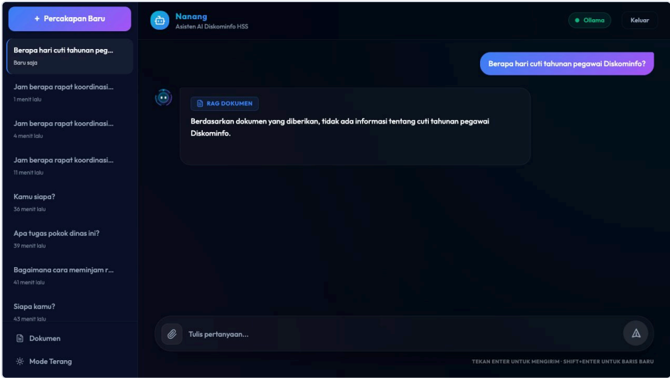
Gambar 7a. Pertanyaan cuti: model tidak mengarang dan sumber tidak ditampilkan.
