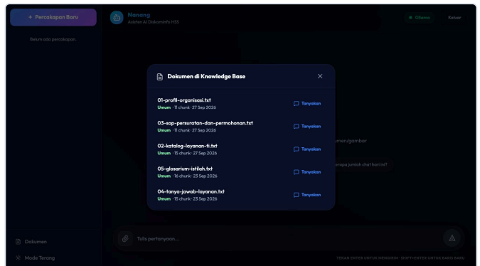
Gambar 5d. Panel Dokumen untuk akun read_only: hanya 5 dokumen Umum, tanpa tombol hapus.
