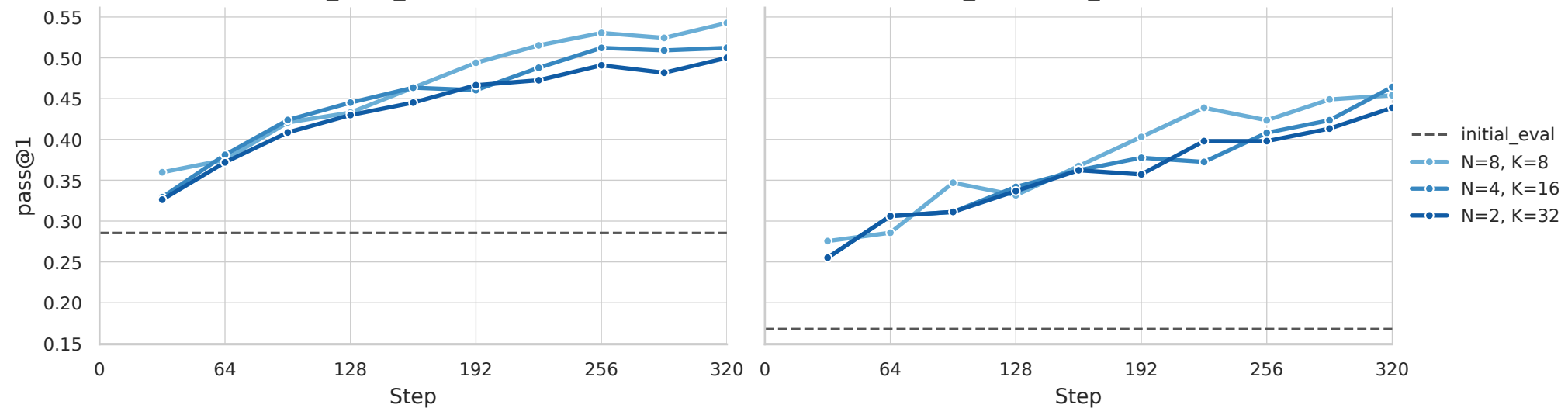
code_stdio_lcbv6 (n=82)
