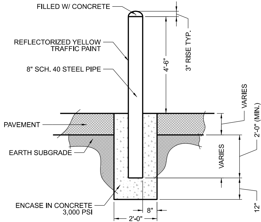
BOLLARD SCALE: 3/8"=1'-0"
