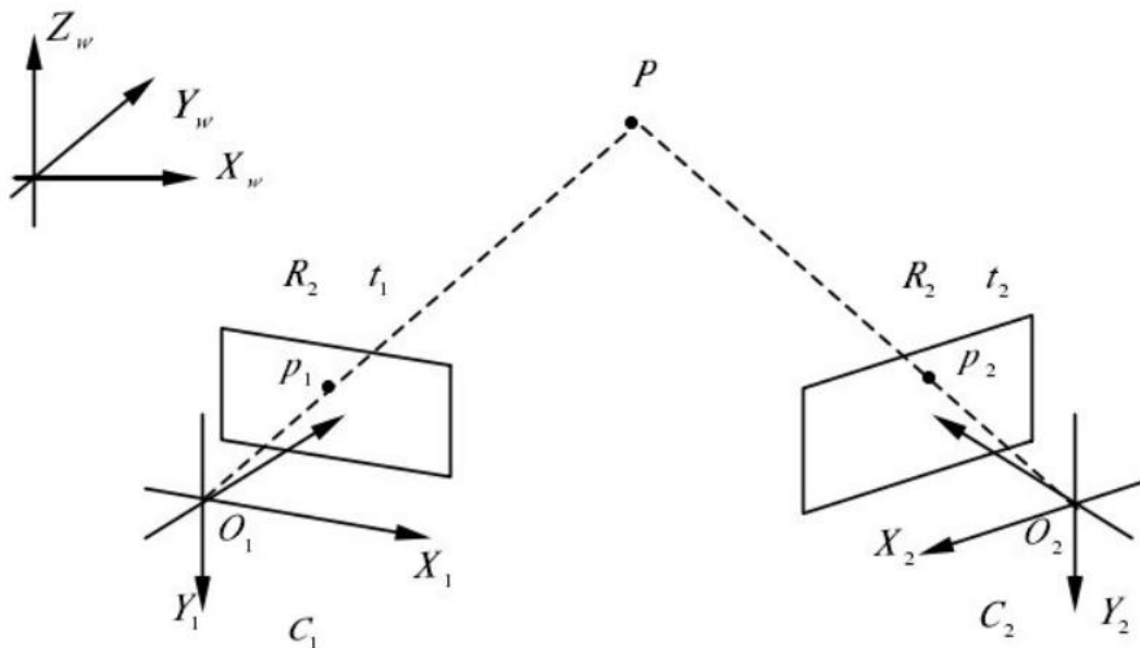
图 12 两部相机拍摄物体 P
