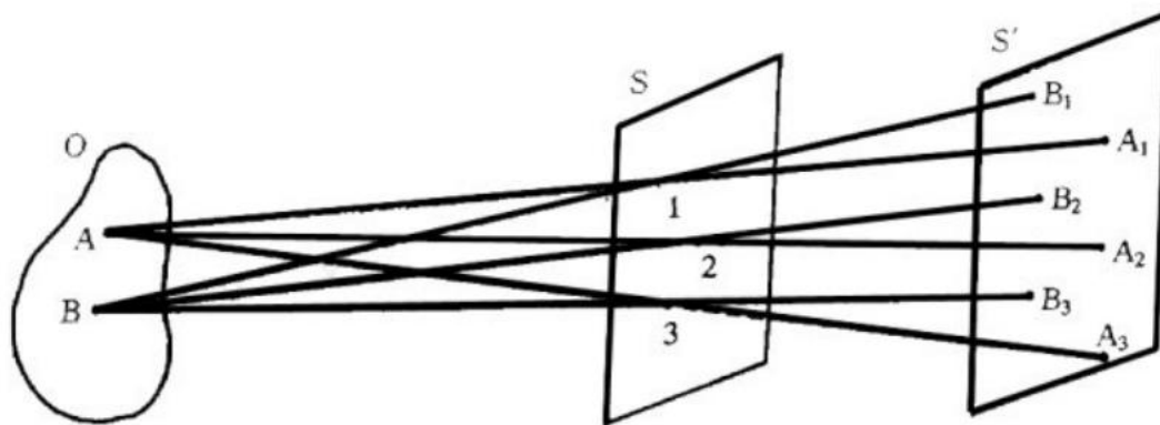
图 3 小孔成像
