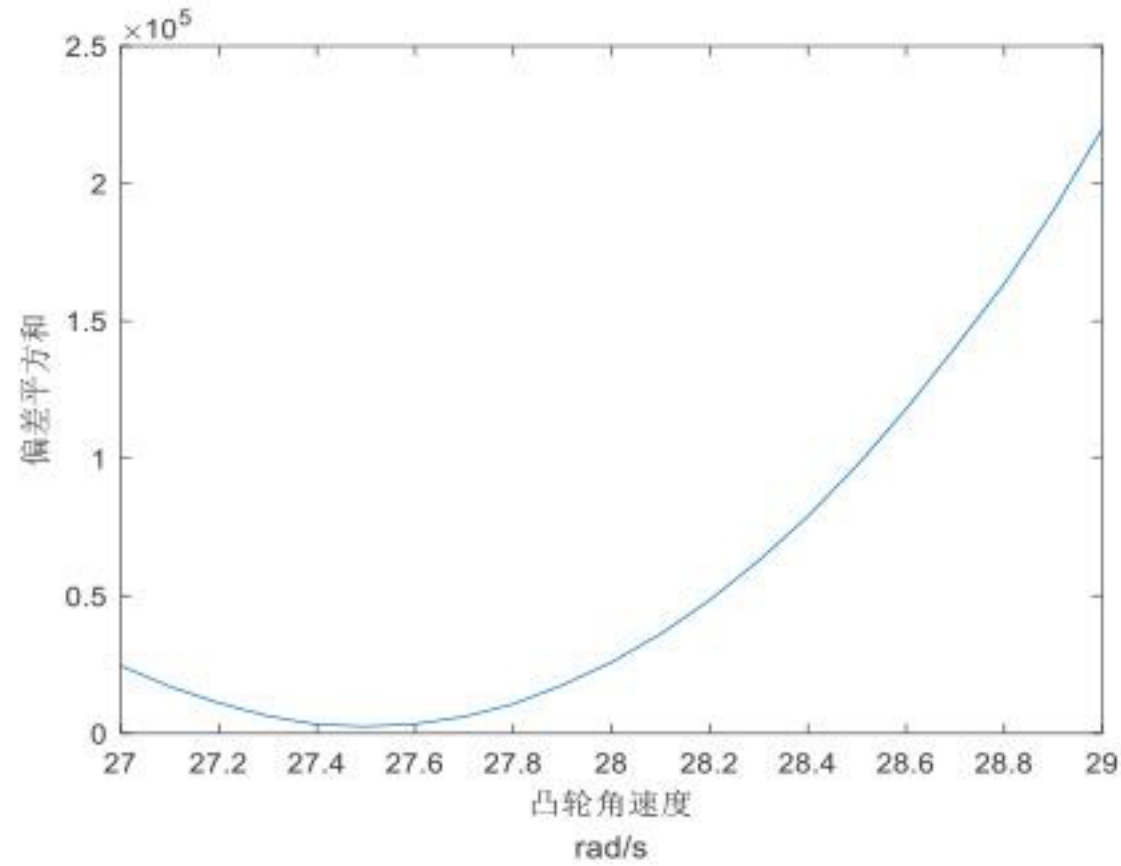
图 20 \omega = 27:29rad/s , 偏差平方和随角速度的变化
