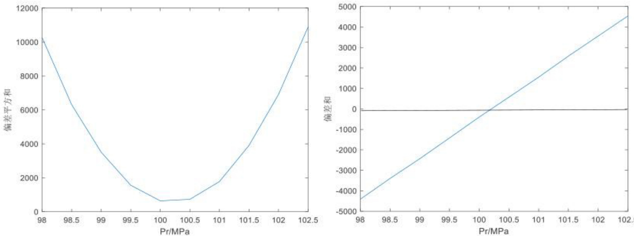
图31、32 \omega = 440\text{rad/s} ， t'_0 = 50\text{ms} ， P_R 为98-102.5MPa，压力偏差平方和和偏差和
