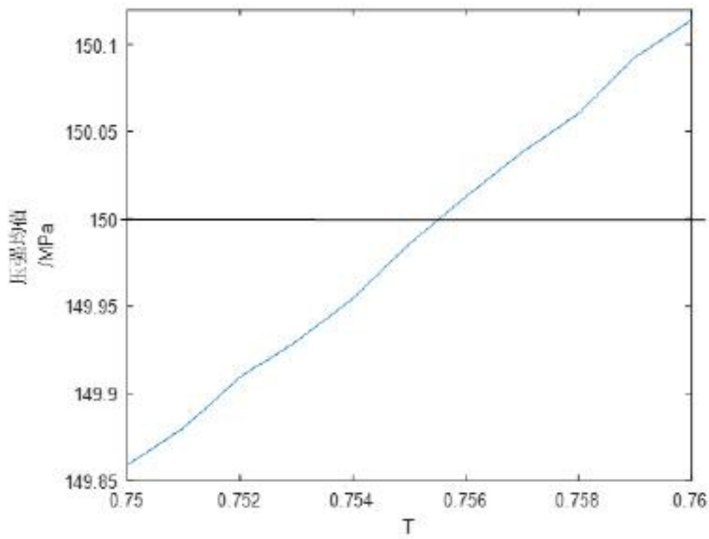
图16 局部放大图
