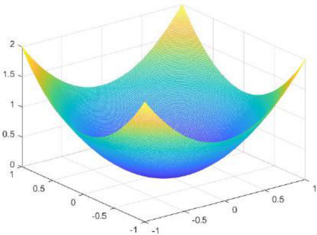
图 24 下凸函数 z = x^2 + y^2 的图像
