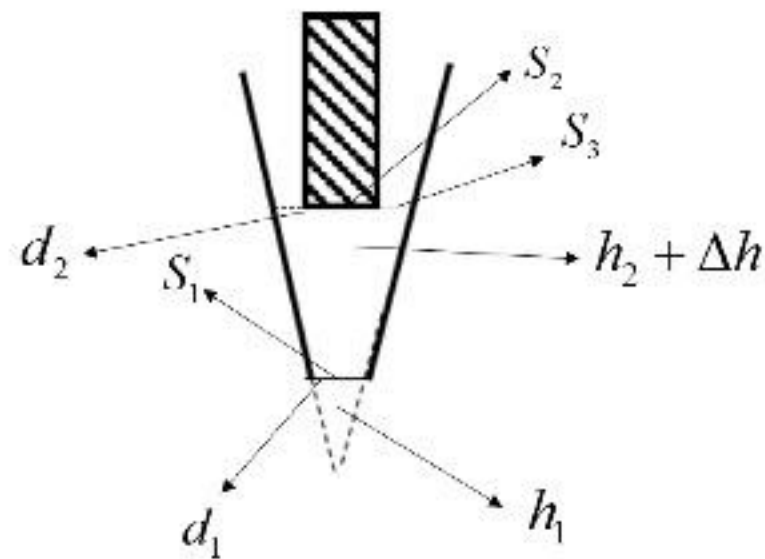
图 17 针阀上升后
