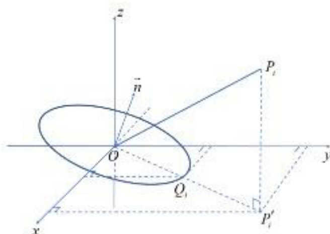
图8 自然坐标系的建立
