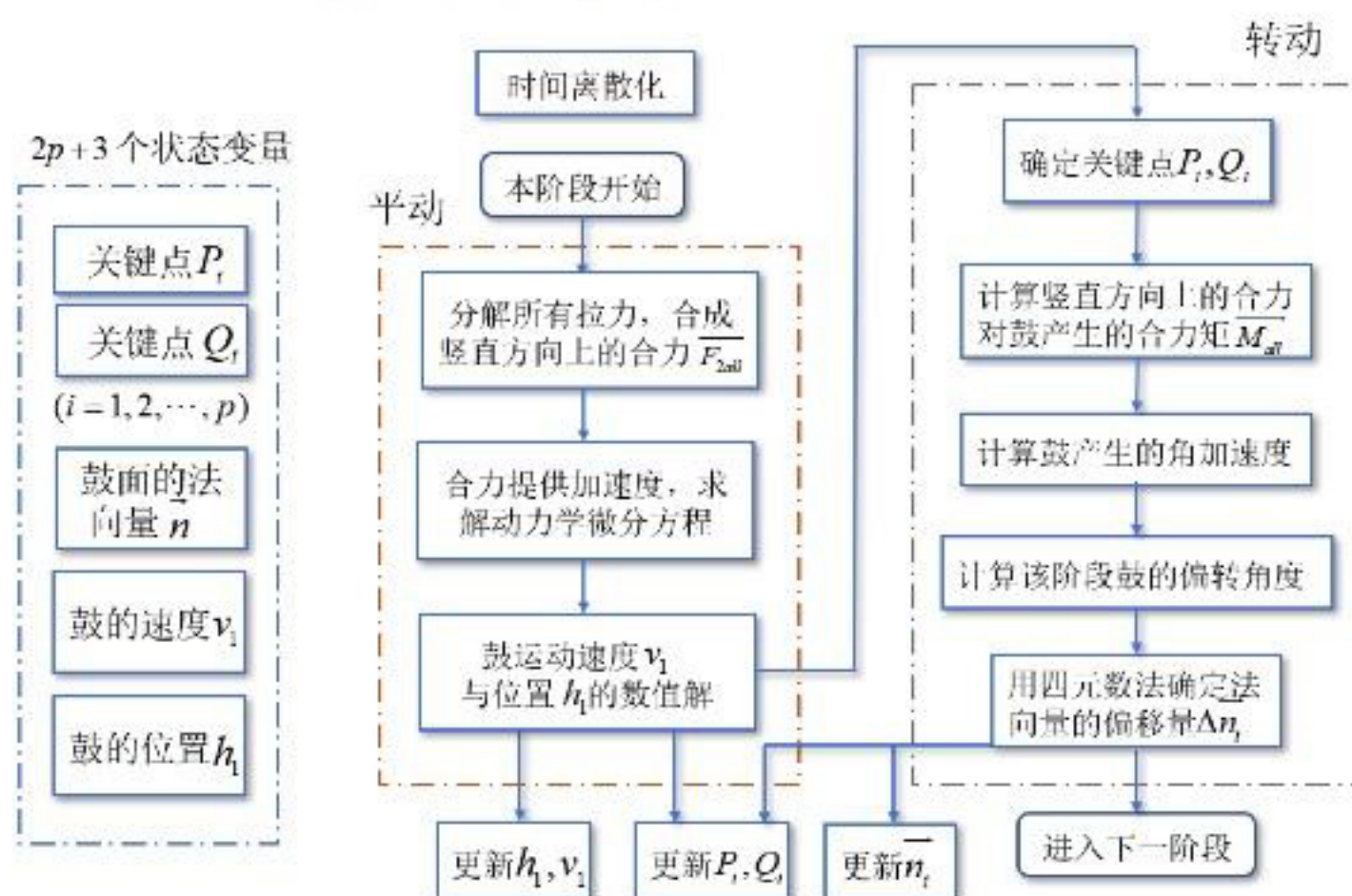
图7 问题二模型框图
