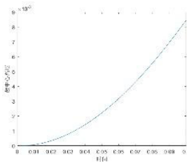
图12 鼓面中心高度随时间变化图示
