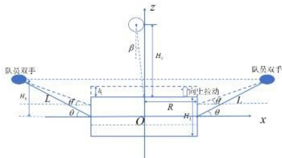
图2 颠球环境变量与坐标系建立示意图
