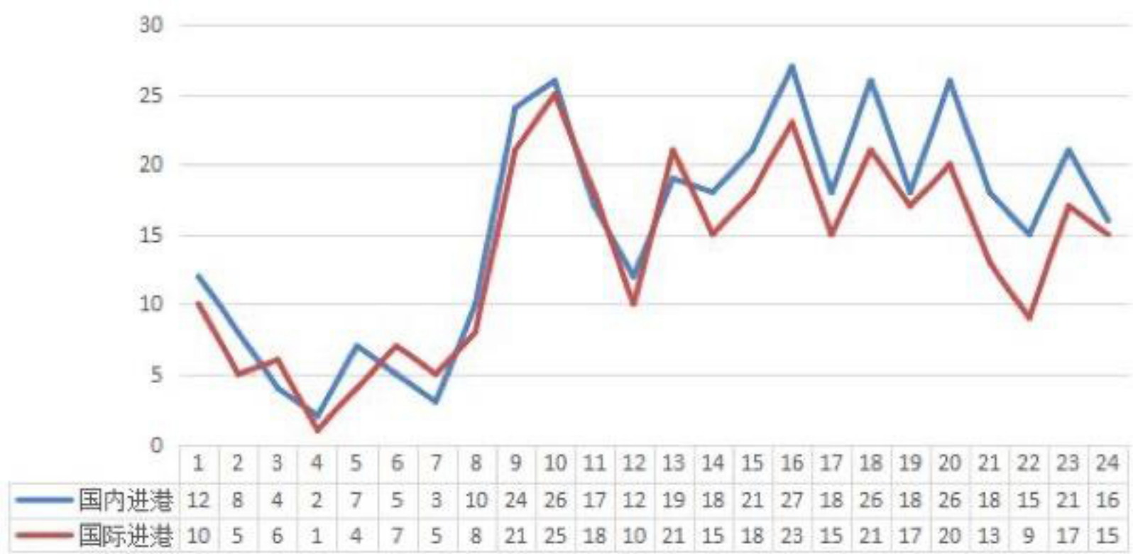
图 4-1 部分机场各时段平均入港飞机架次分布规律
