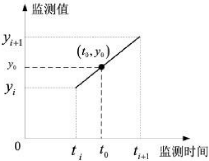
图 6 线性插值
