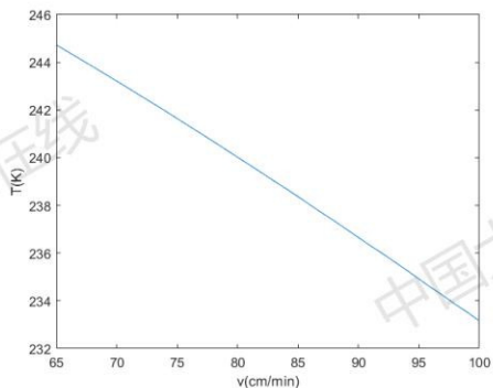
图 15: 峰值温度随过炉速度变化曲线
