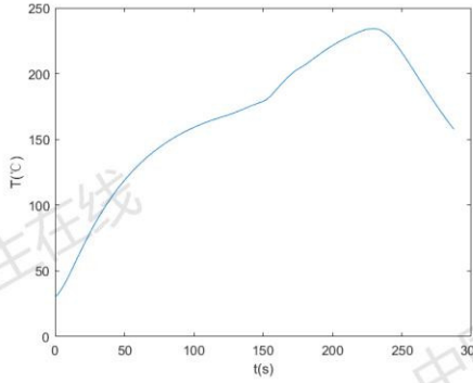
图 20: 问题四炉温曲线
