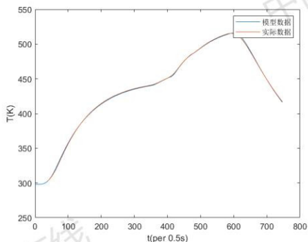
图 8: 实验炉温曲线对比
