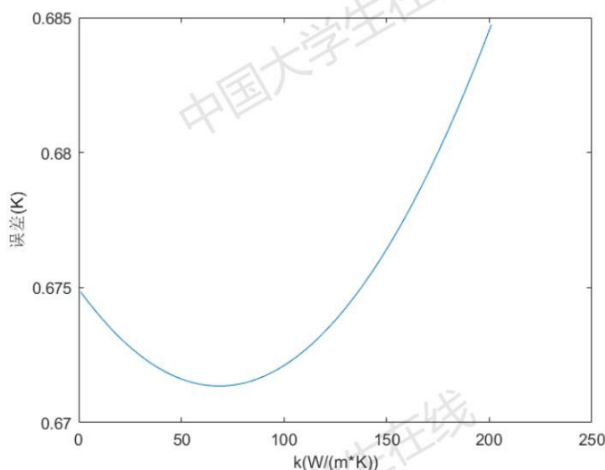
图 7: 均方根误差变化曲线
