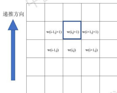
图 6: 有限差分法解偏微分方程示意图
