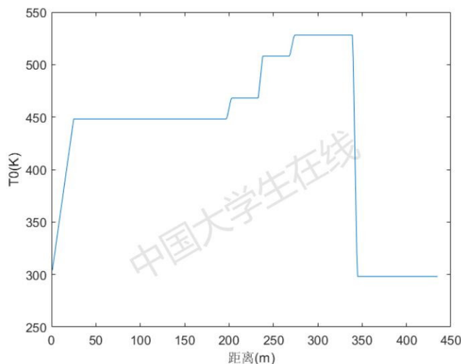
图 5: 实验中的环境温度
