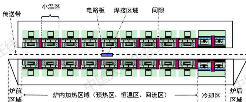
图 1: 回焊炉截面示意图
