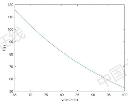
图 13: 升温时 150^{\circ}\text{C} \sim 190^{\circ}\text{C} 时间与速度关系
