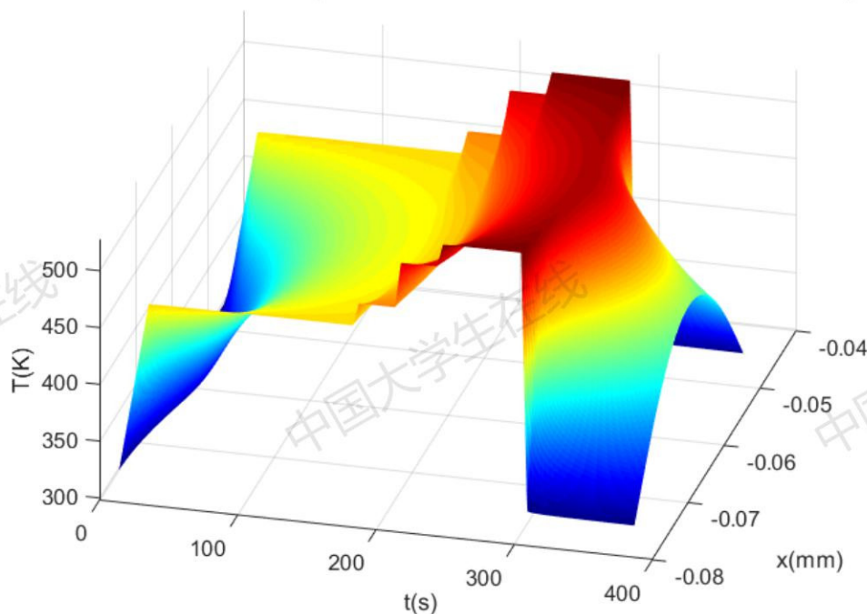
图 11: 温度分布伪彩图
