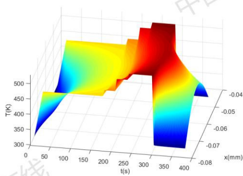
图 9: 工件整体温度分布
