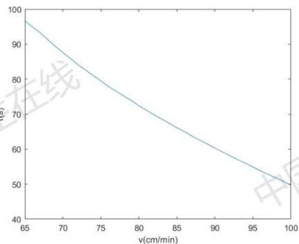
图 14: 温度大于 217^{\circ}\text{C} 时间随速度变化曲线
