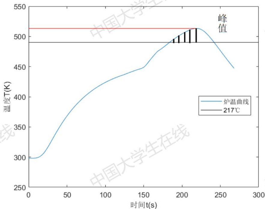
图 18: 最优解炉温曲线
