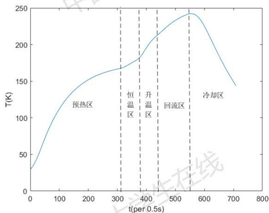
图 2: 实际炉温曲线
