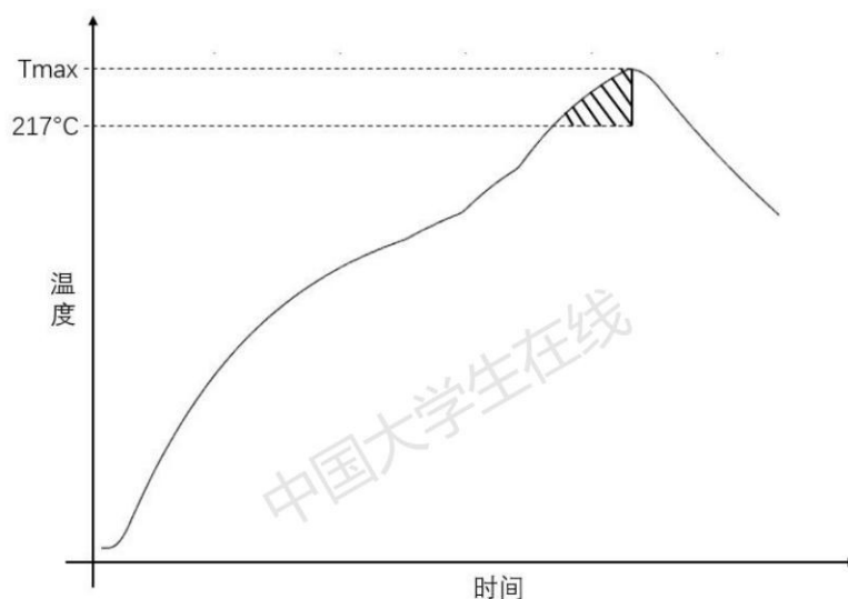
图 7、峰值温度覆盖面积示意图
