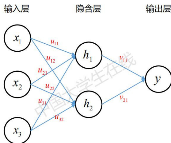
图 6.5 BP 神经网络传播图
