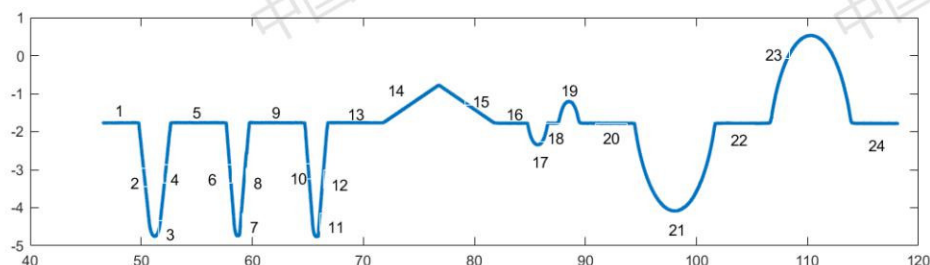
图 5.1.1-1 工件 1 轮廓散点图
