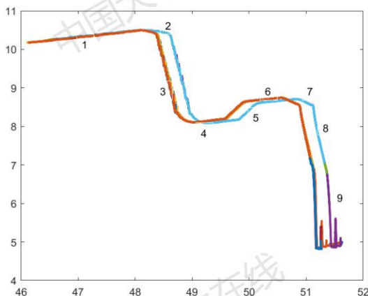
图 5.4.2-1 9 个数据的轮廓重合图
