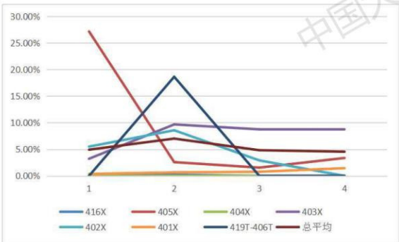
图 14、各子网漏损比率随季度走势图（2σ）图 15、各子网漏损比率随季度走势图（3σ）
