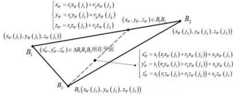
图 9: 反馈面板三角形区域示意图
