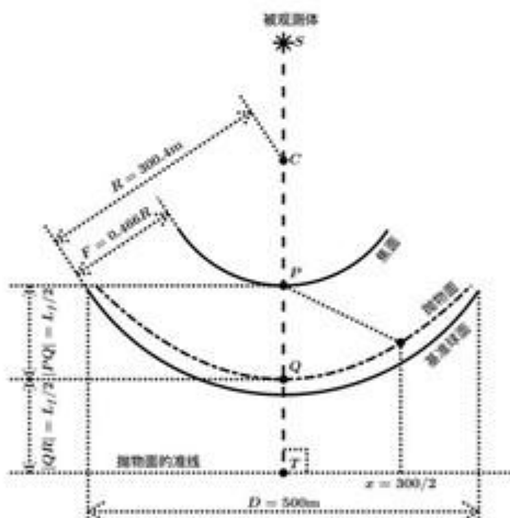
图 1: FAST 剖面示意图
