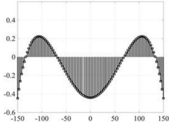
图 5：最优抛物面与基准球面的偏移量
