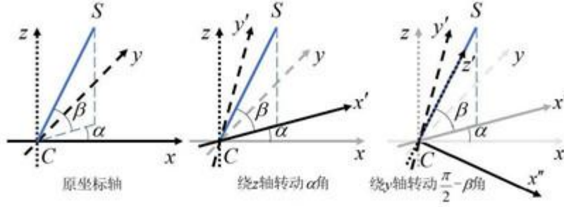
图 6: 坐标系旋转示意图
