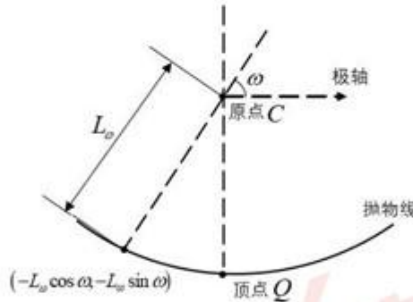
图 2：极坐标系下抛物线示意图
