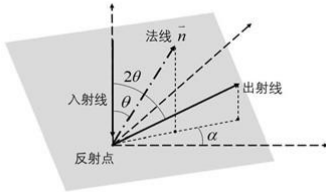
图 10: 各角度三维示意图
