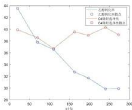
图 4 乙醇转化率与 C4 选择性散点图
