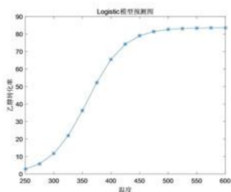
图 2 B1 组的乙醇转化率趋势预测图
