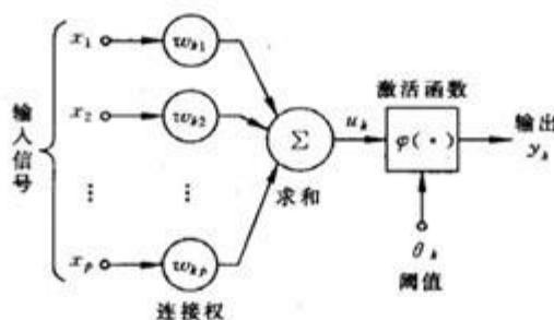
图 5.4-1：人工神经网络基本单元的神经模型
