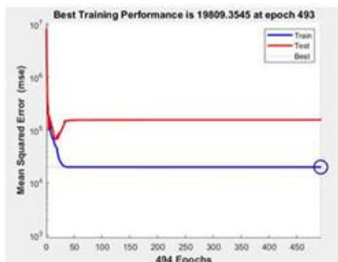
图 5.4-3: 第 493 代时最优训练效果
