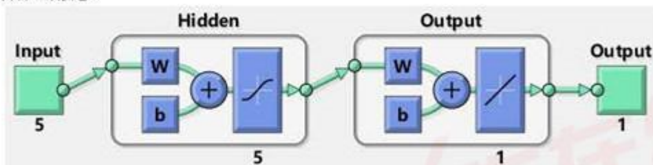
图 5.4-2：针对该问题的 5 个输入 5 个神经元的 BP 神经网络模型
