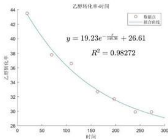
图 5.2-1 乙醇转化率随时间呈指数衰减特征
