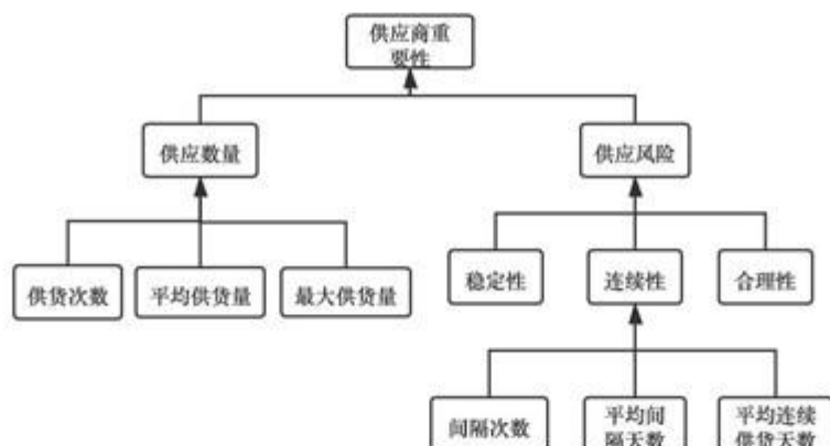
图 1：问题一多指标评价模型
