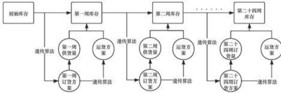
图 2: 问题二的多目标规划模型
