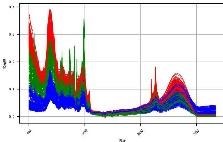
图 5 附件 1 分类后光谱曲线图
