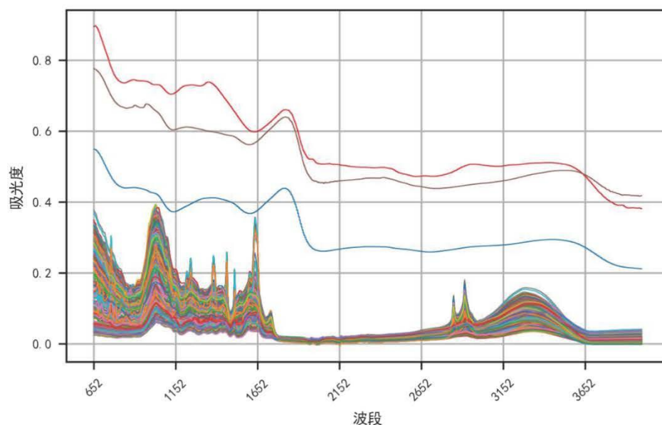
图 1 附件 1 原始数据图
