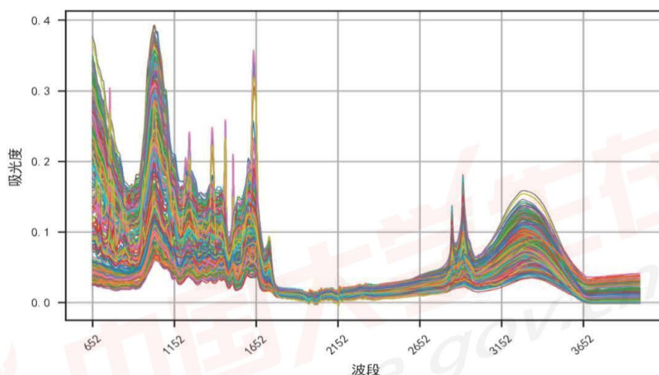
图 2 附件 1 删除原始数据后的图
