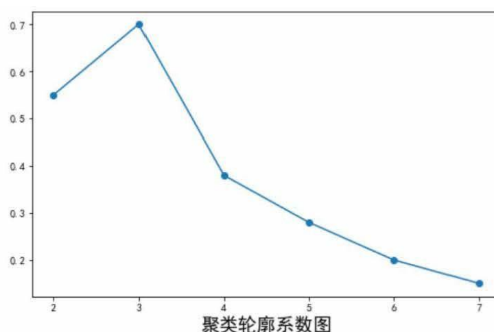
图 4 K-means 聚类轮廓系数
