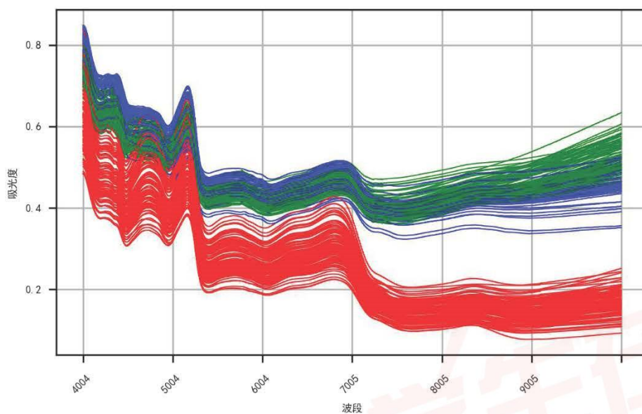
图 11 附件 4 按不同类别着色的数据图
