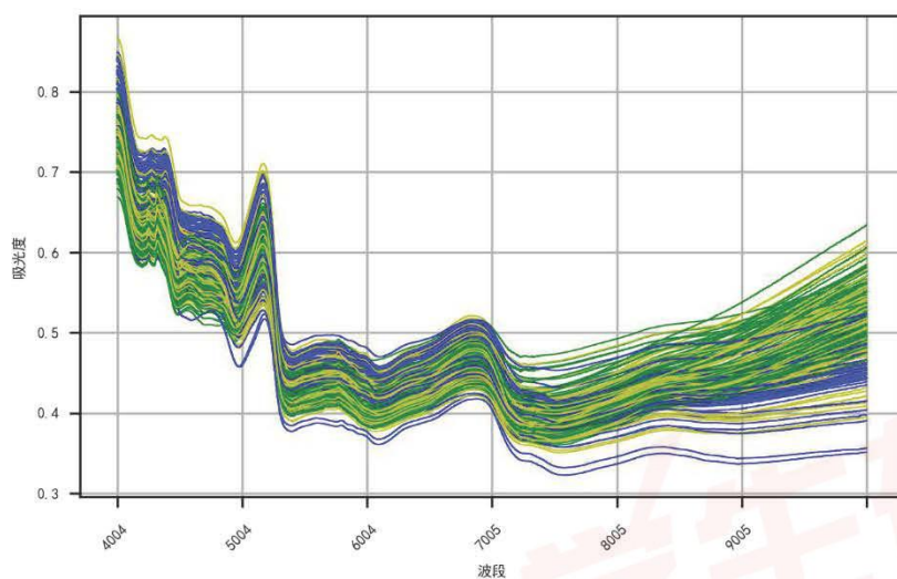
图 13 附件 4 中 BC 类数据及未分类数据图
