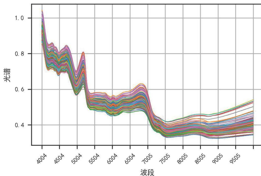
图 10 附件 3 近红外原始数据
