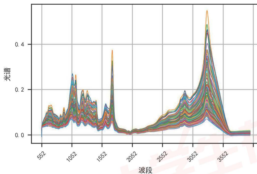
图 9 附件 3 中红外原始数据
