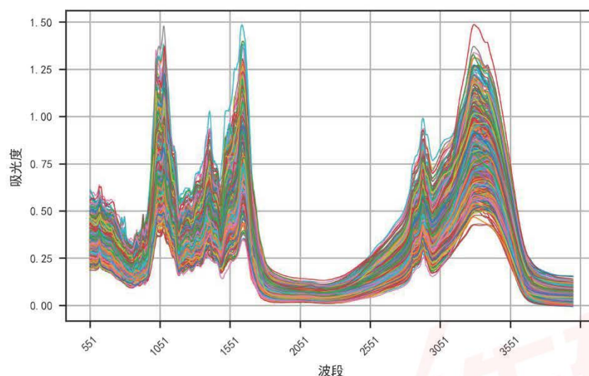
图 6 附件 2 原始数据图
