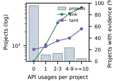
(d) API-volume strata
