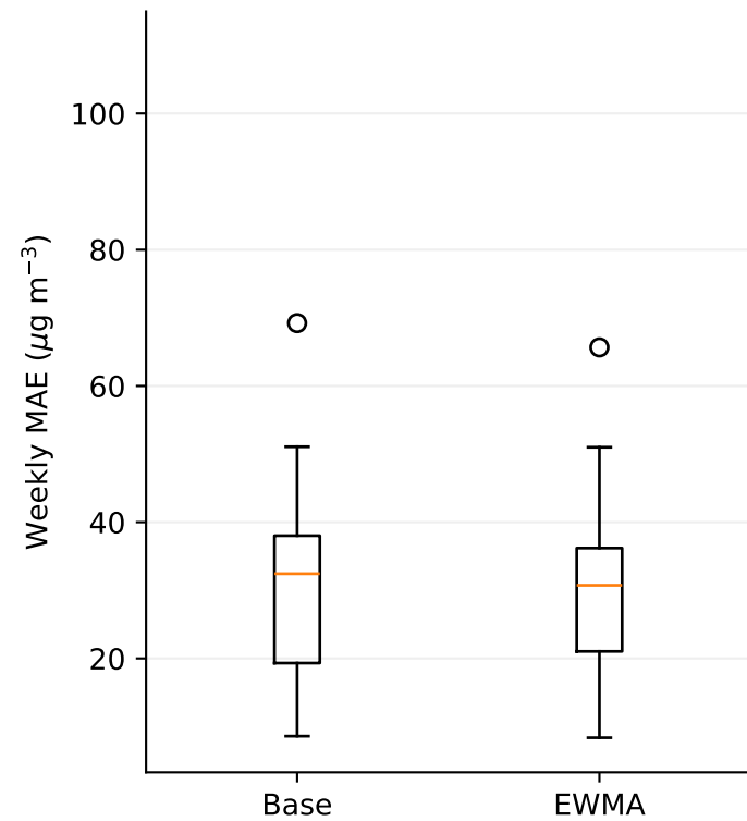
SARIMAX
