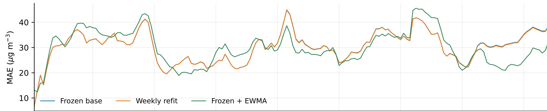
SARIMAX
