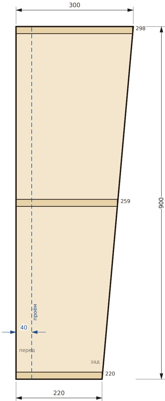
Вид слева: боковина и разделители
