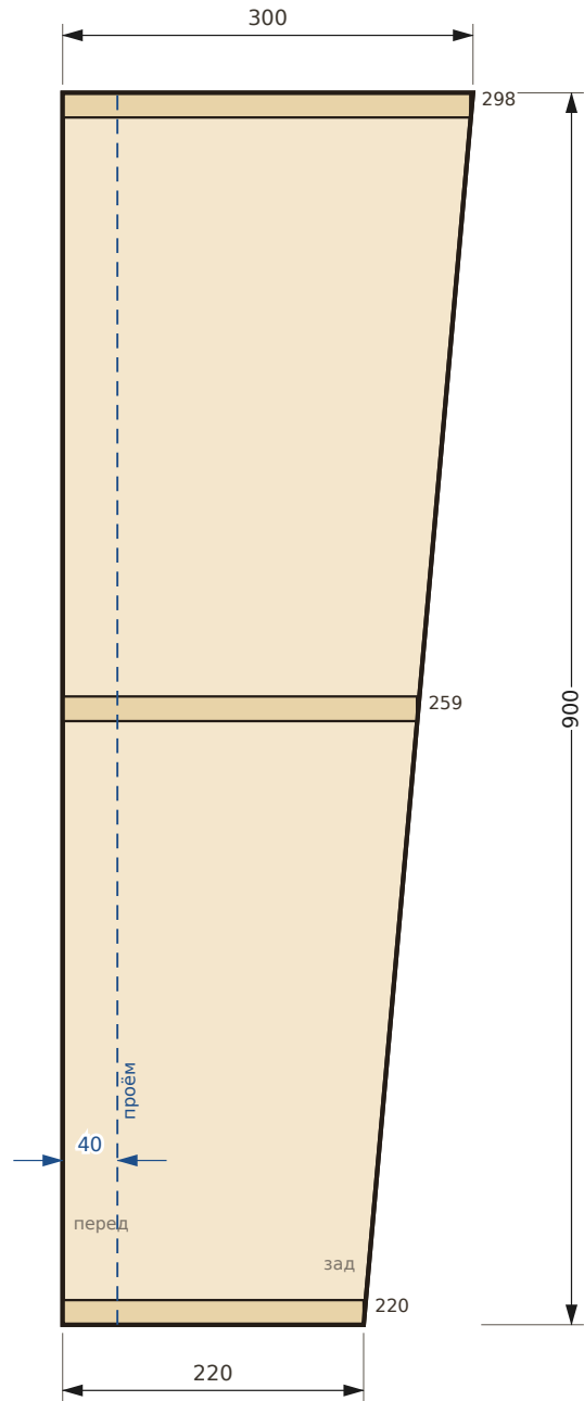
Вид слева: боковина и разделители
