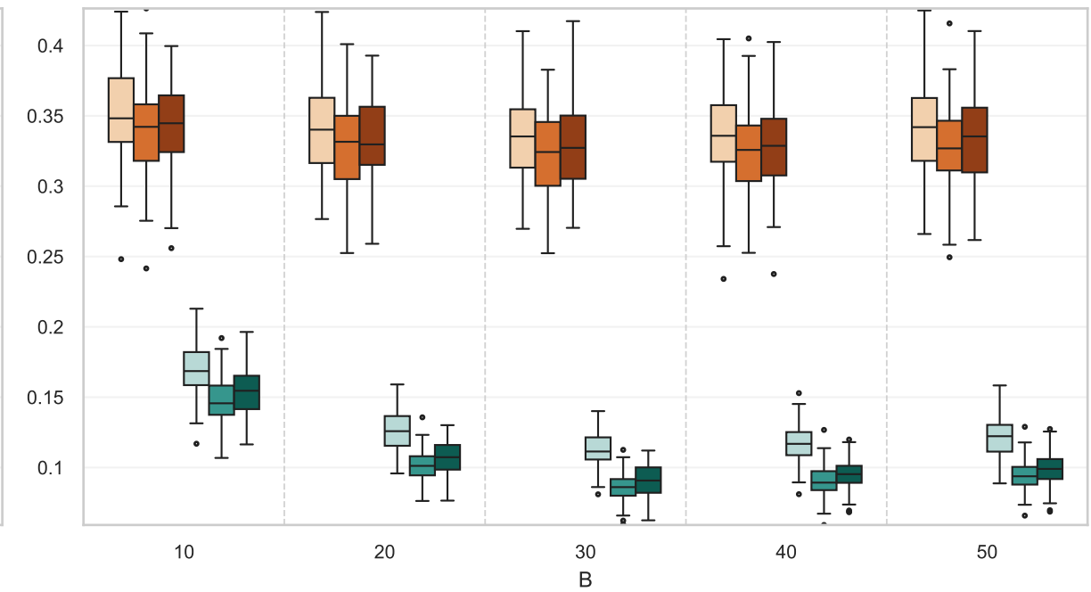
(d) Forecast | Nonlinear
