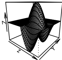
True persp
