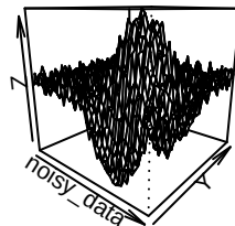
Noisy persp
