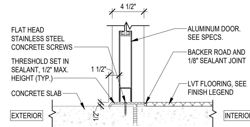
9 DOOR SILL - ALUMINUM DOOR A-602 SCALE: 1 1/2" = 1'-0"
