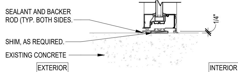
12 WINDOW SILL A-602 SCALE: 1 1/2" = 1'-0"
