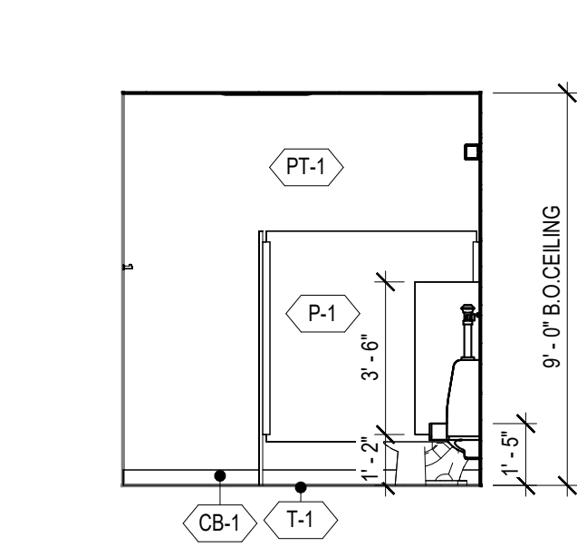
4 A-112 MENS RESTROOM SCALE: 1/4" = 1'-0"
