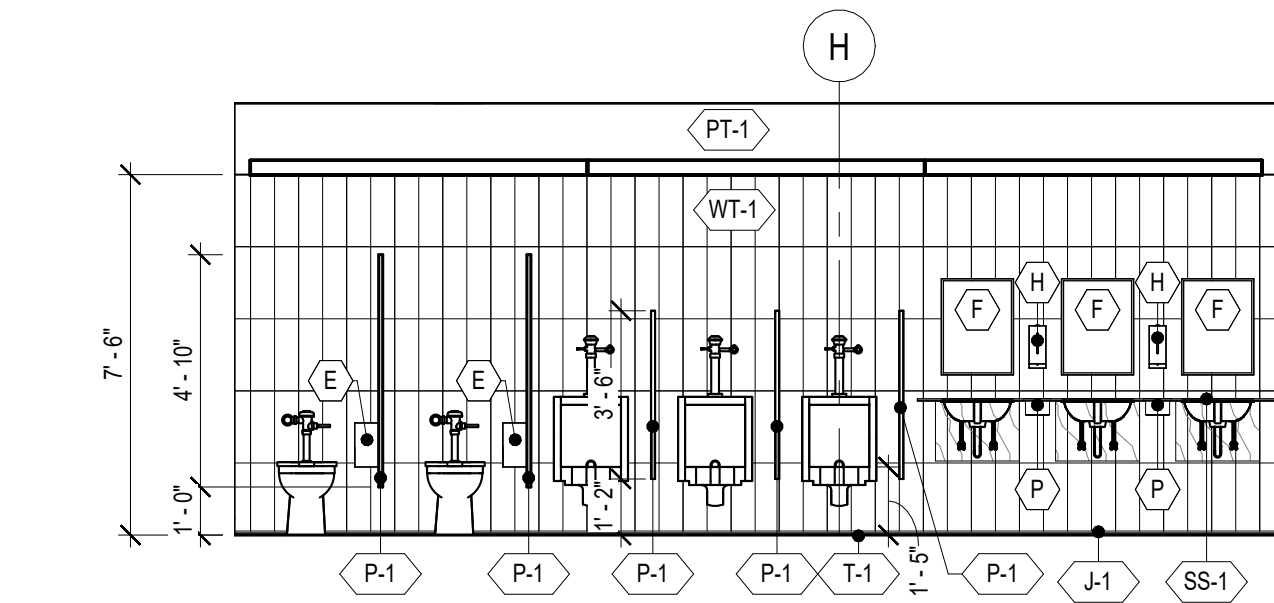
1 A-112 MENS RESTROOM SCALE: 1/4" = 1'-0"
