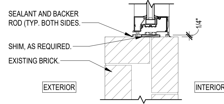
13 WINDOW JAMB A-602 SCALE: 1 1/2" = 1'-0"
