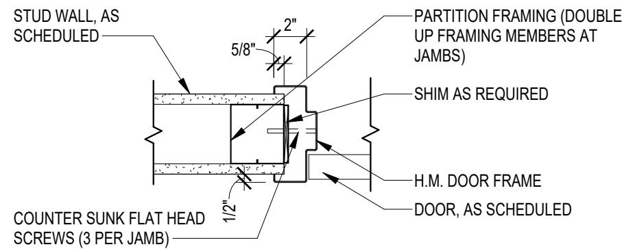
5 DOOR JAMB - HM DOOR @ GWB A-602 SCALE: 1 1/2" = 1'-0"
