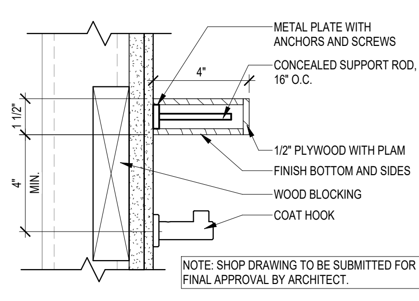
5 A-112 SHELF DETAIL SCALE: 3" = 1'-0"
