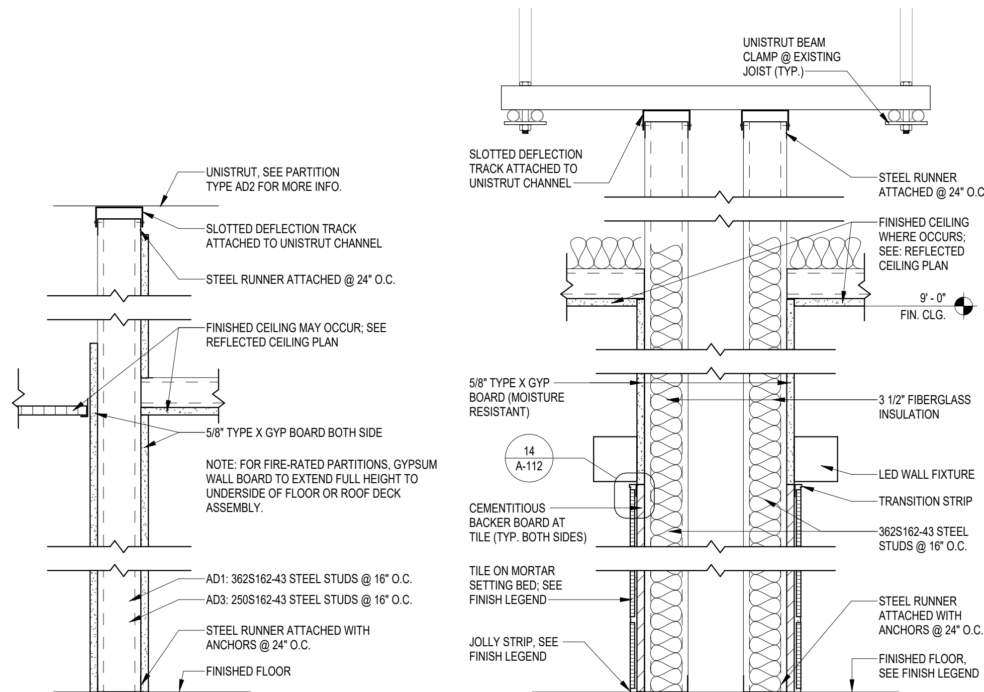
11 A-112 PARTITION TYPE AD1/AD3 SCALE: 1 1/2" = 1'-0"
