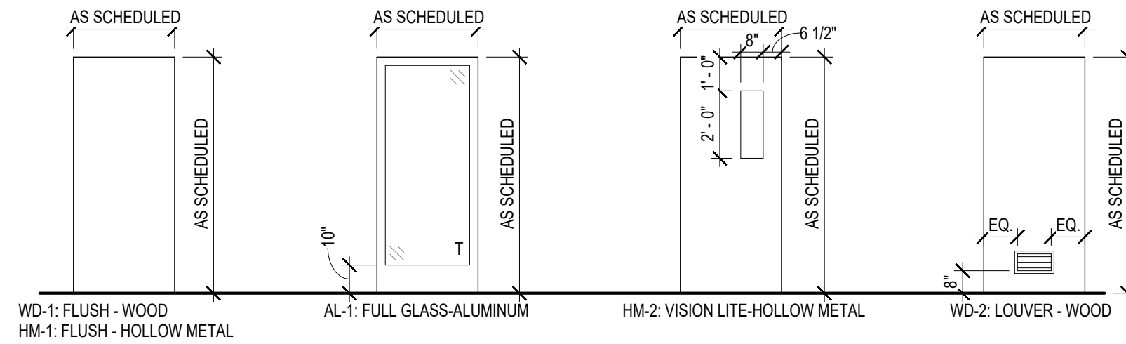
1 DOOR TYPES A-602 SCALE: 1/4" = 1'-0"
