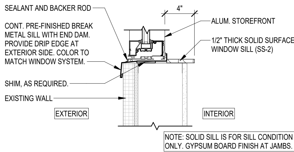
11 WINDOW SILL A-602 SCALE: 1 1/2" = 1'-0"
