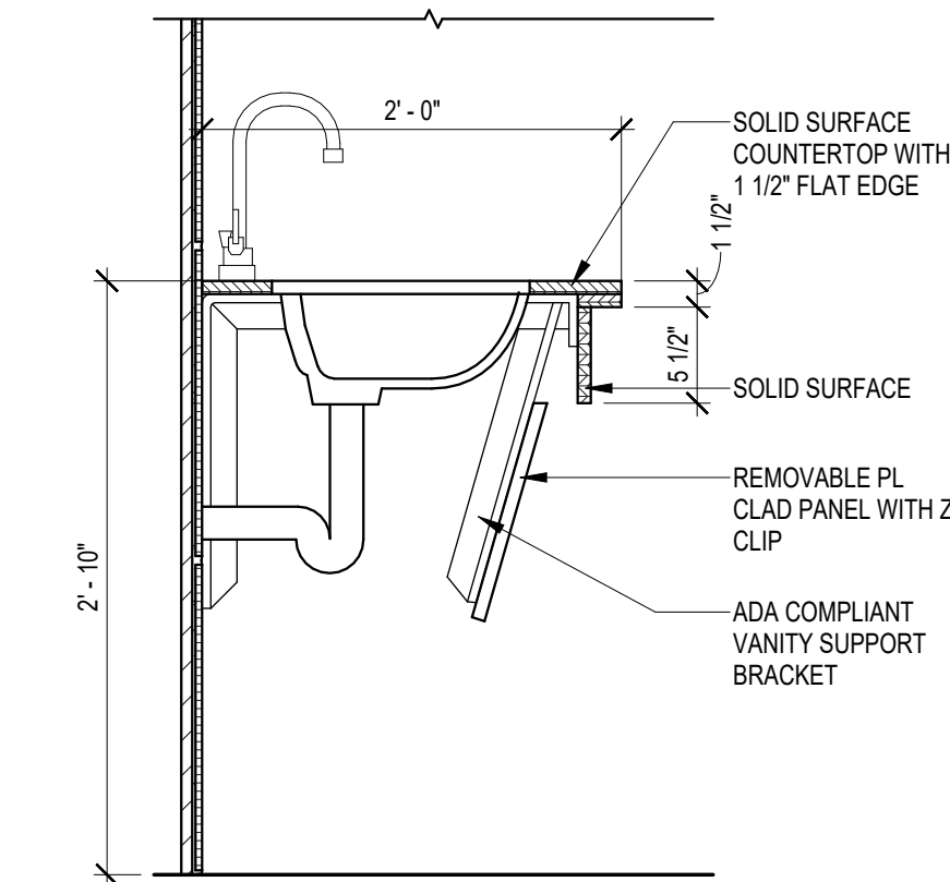
10 A-112 TYP. LAV BASE CAB SCALE: 1" = 1'-0"
