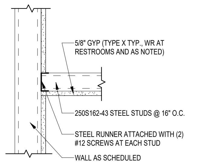
13 A-112 GYPSUM CEILING SCALE: 1 1/2" = 1'-0"
