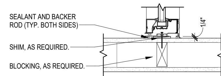
14 WINDOW JAMB A-602 SCALE: 1 1/2" = 1'-0"
