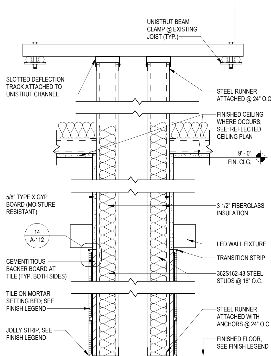
12 A-112 PARTITION TYPE AD2 SCALE: 1 1/2" = 1'-0"
