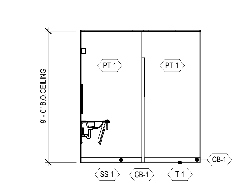
2 A-112 MENS RESTROOM SCALE: 1/4" = 1'-0"
