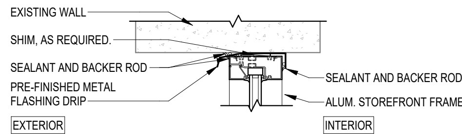
10 WINDOW HEAD A-602 SCALE: 1 1/2" = 1'-0"
