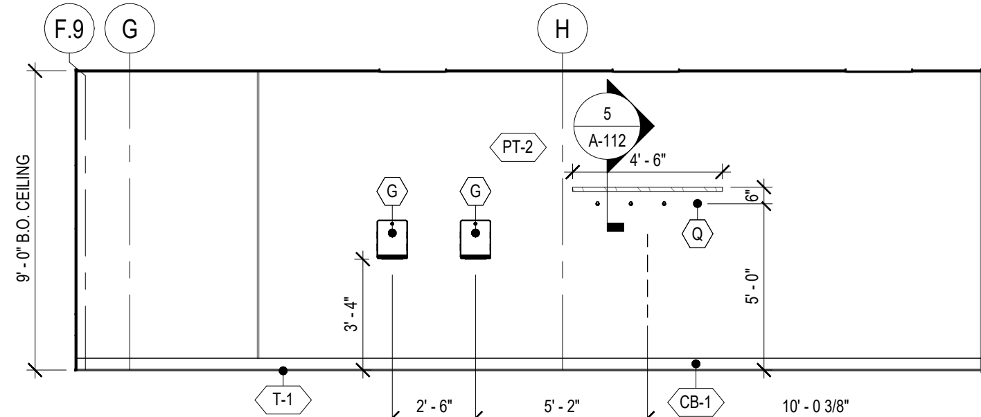
3 A-112 MENS RESTROOM SCALE: 1/4" = 1'-0"
