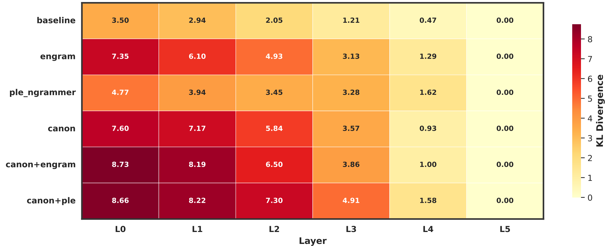
LogitLens KL Divergence
