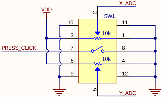
JOYSTICK
