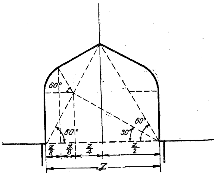
Рис. 48. Схема построения арки в мечети Намазгох.
