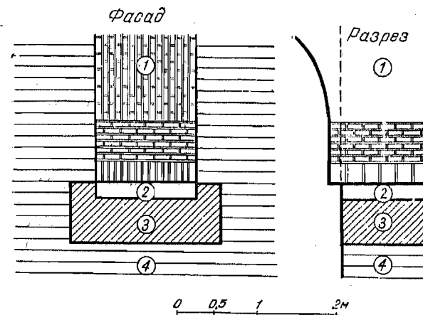
Рис. 9. Конструкция опоры арки из жженого кирпича на сырцовую стену в мечети Диггарон:
