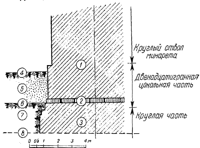
Рис. 46. Фундаменты Бабкентского минарета:
