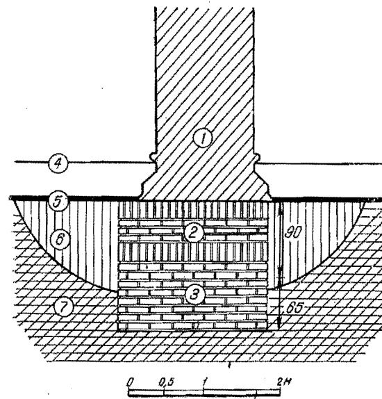
Рис. 44. Фундаменты колонн мечети в Хазаре (Диггарон):
