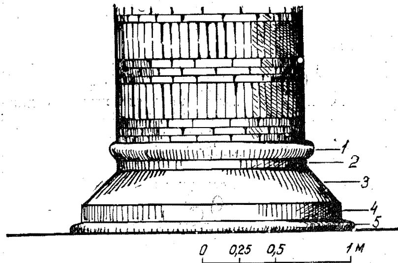
Рис. 8. Нижняя часть колонны в мечети Диггарон: 1—поджатый книзу валик; 2—продолжение ствола колонны; 3—конический раструб; 4—цилиндр; 5—приплюснутый вал.
