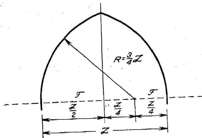
Рис. 47. Схема построения арки в мавзолеев Мир-сеид-Бахром.
