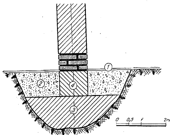
Рис. 45. Фундаменты стен мечети Магор-и Аттари: 1—уровень земли XII в.; 2—рыхлая засыпка; 3—основание из кирпичного щебня на глиняном растворе; 4—фундамент из жженого кирпича на алебастровом растворе.
