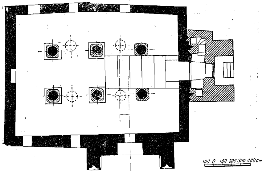
Рис. 31. План мечети Магок-и Аттари (пунктиром показаны колонны X в.).
