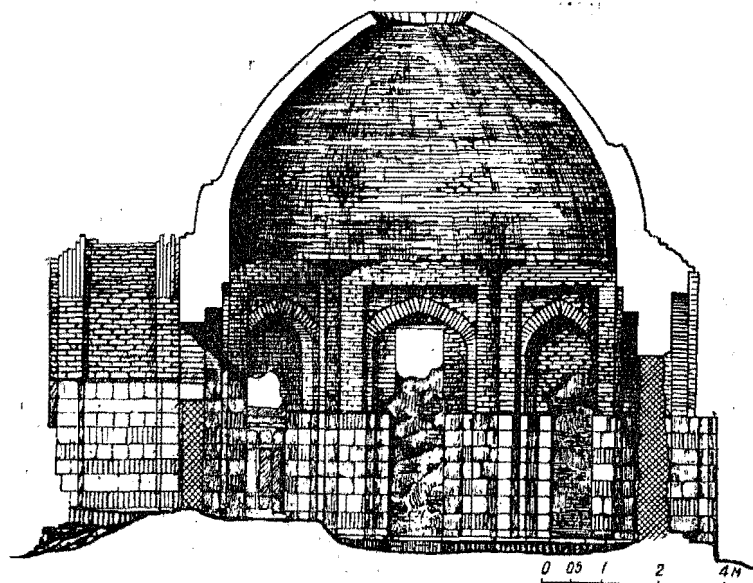
Рис. 23. Шабурган-ата. Разрез здания по главной оси.
