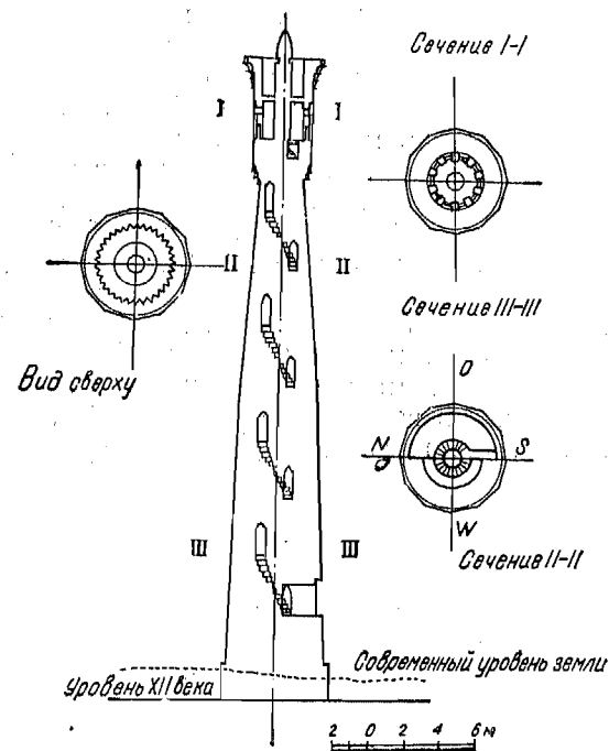
Рис. 43. Разрез и плановые сечения Вабкентского минарета.
