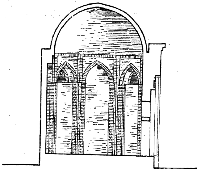
Рис. 12. Мавзолей Мир-сеид-Бахром. Разрез по главной оси.
