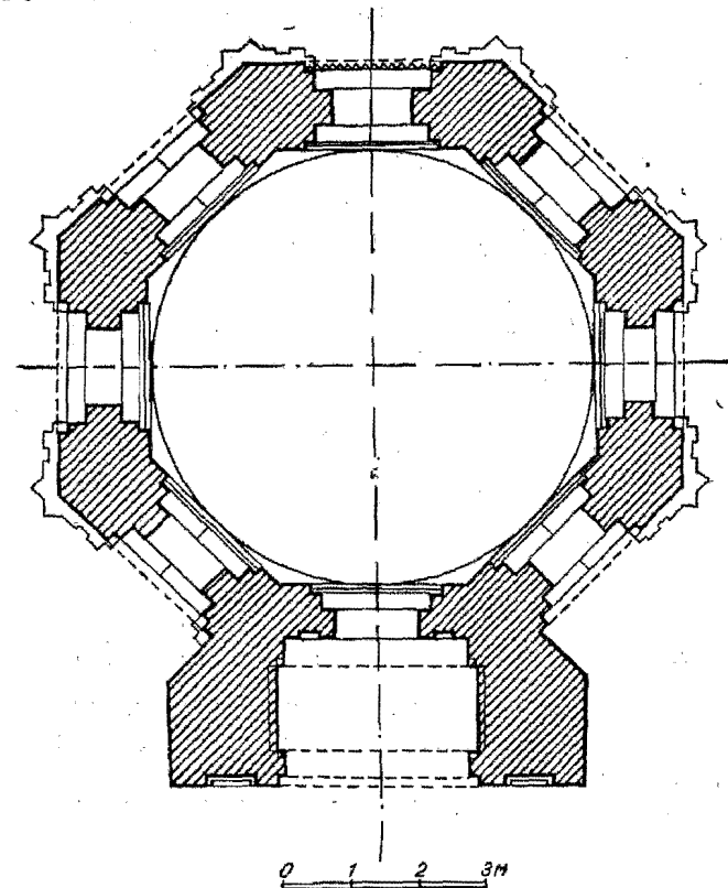
Рис. 22. План здания Шабурган-ата (с реконструкцией разрушенных частей цоколя).
