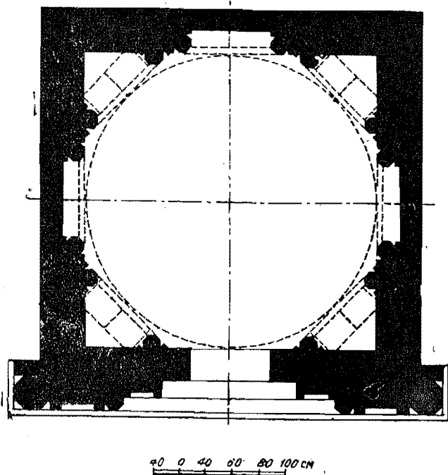
Рис. 11. План мавзолея Мир-сеид-Бахром.
