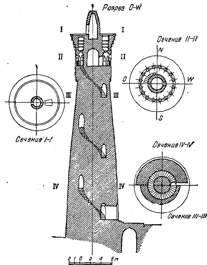
Рис. 36. Разрез и плановые сечения минарета Калаян.
