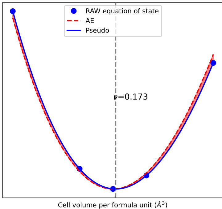
EOS of XO3
