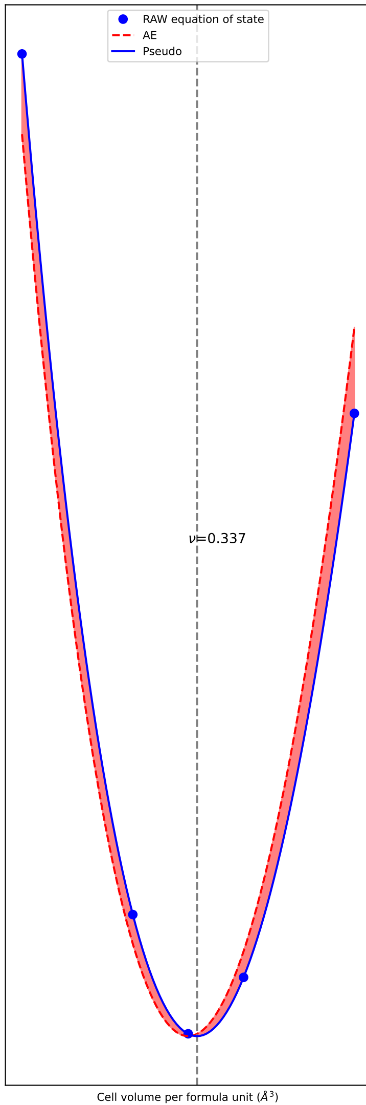
EOS of XO
