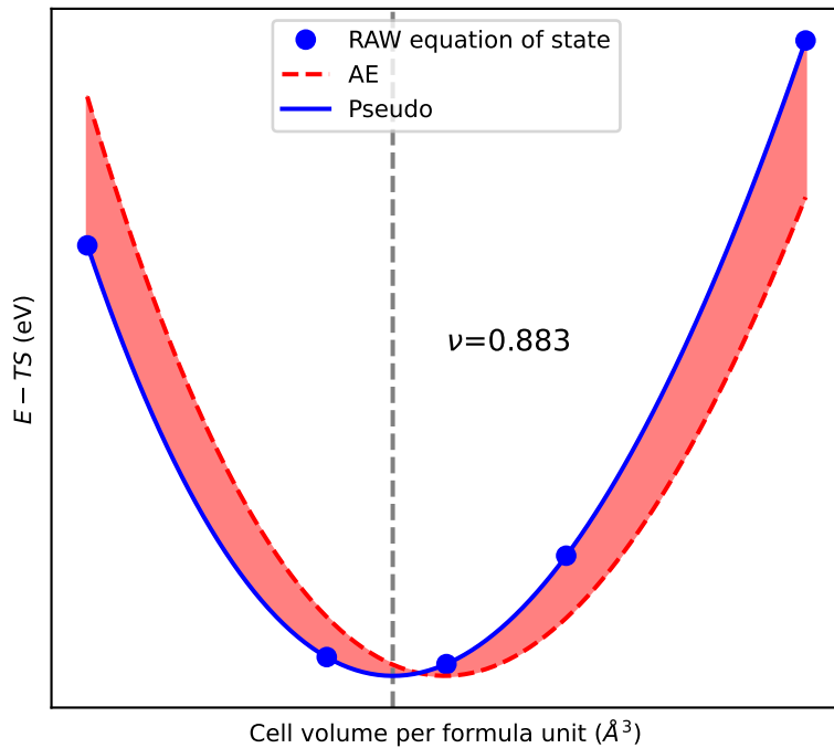
EOS of XO3
