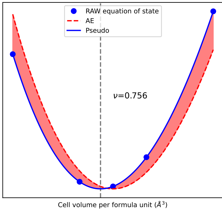
EOS of XO2
