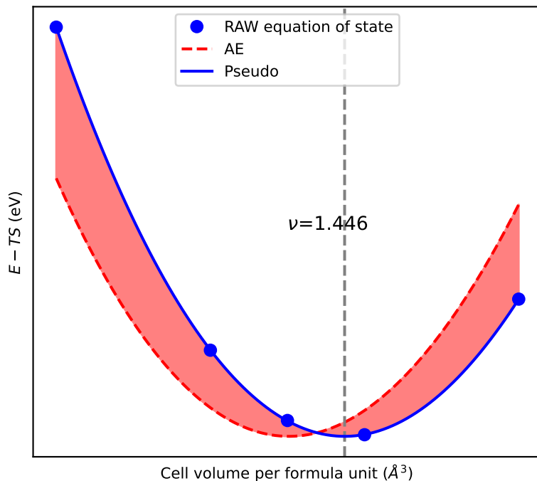
EOS of XO
