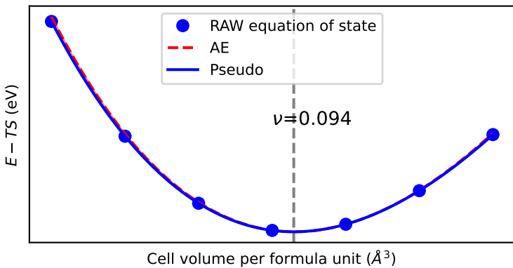
EOS of XO
