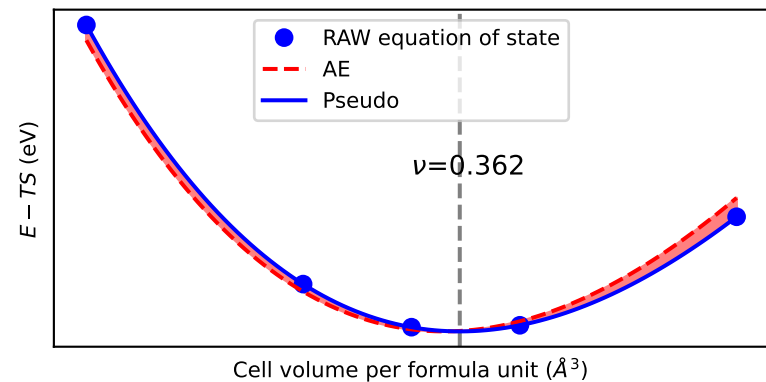
EOS of XO
