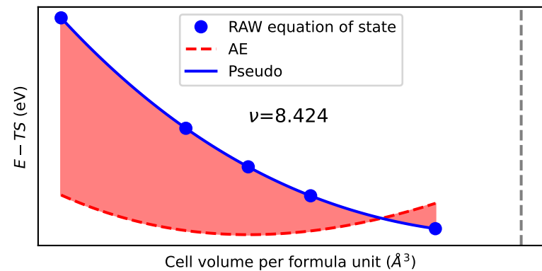
EOS of XO3
