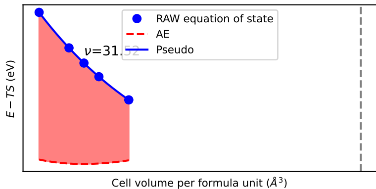
EOS of XO2
