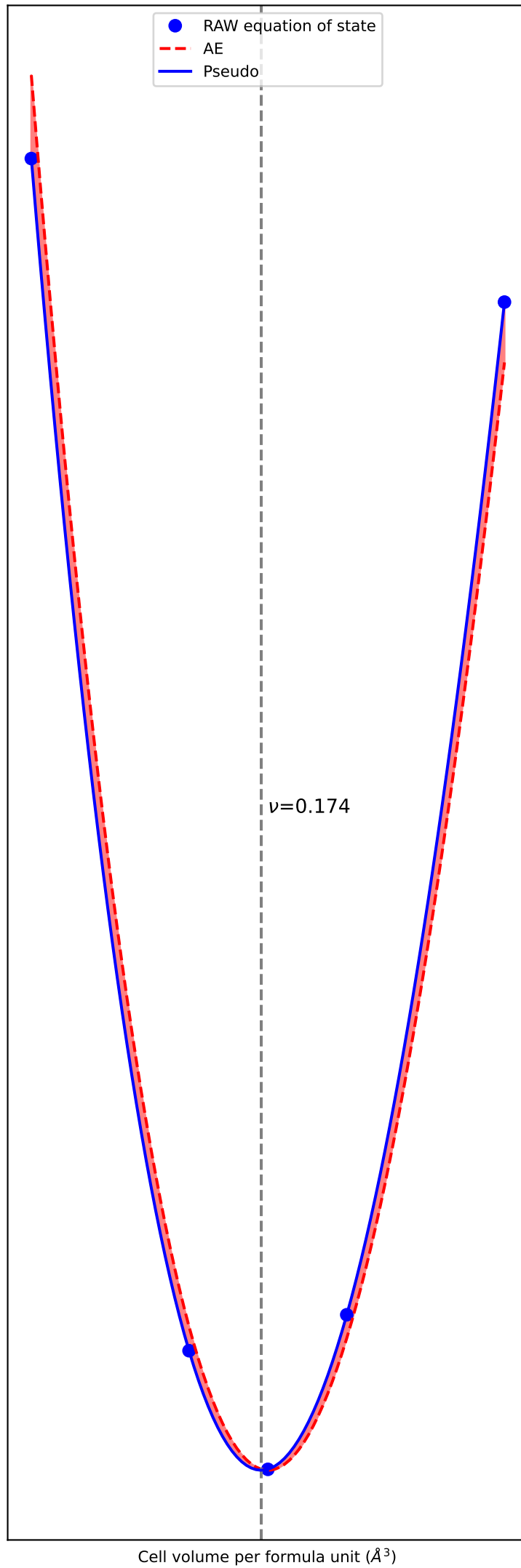
EOS of XO2
