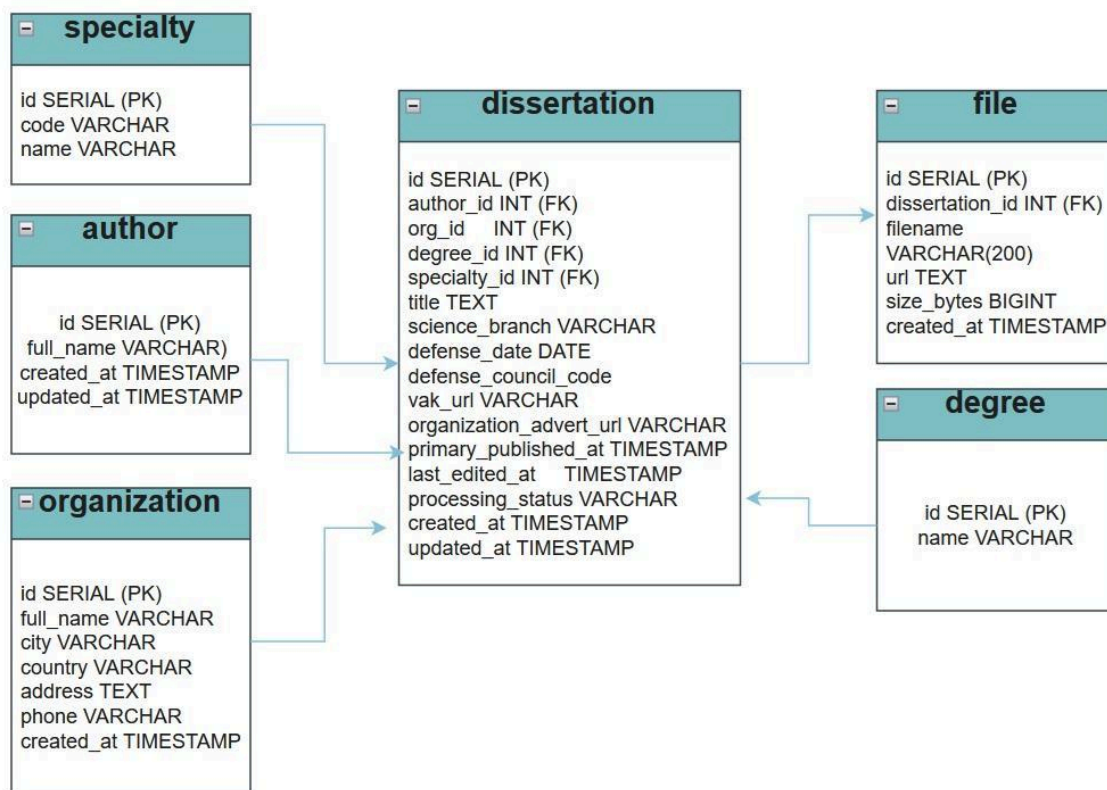
Рисунок 2 - графическое представление реляционной базы данных
