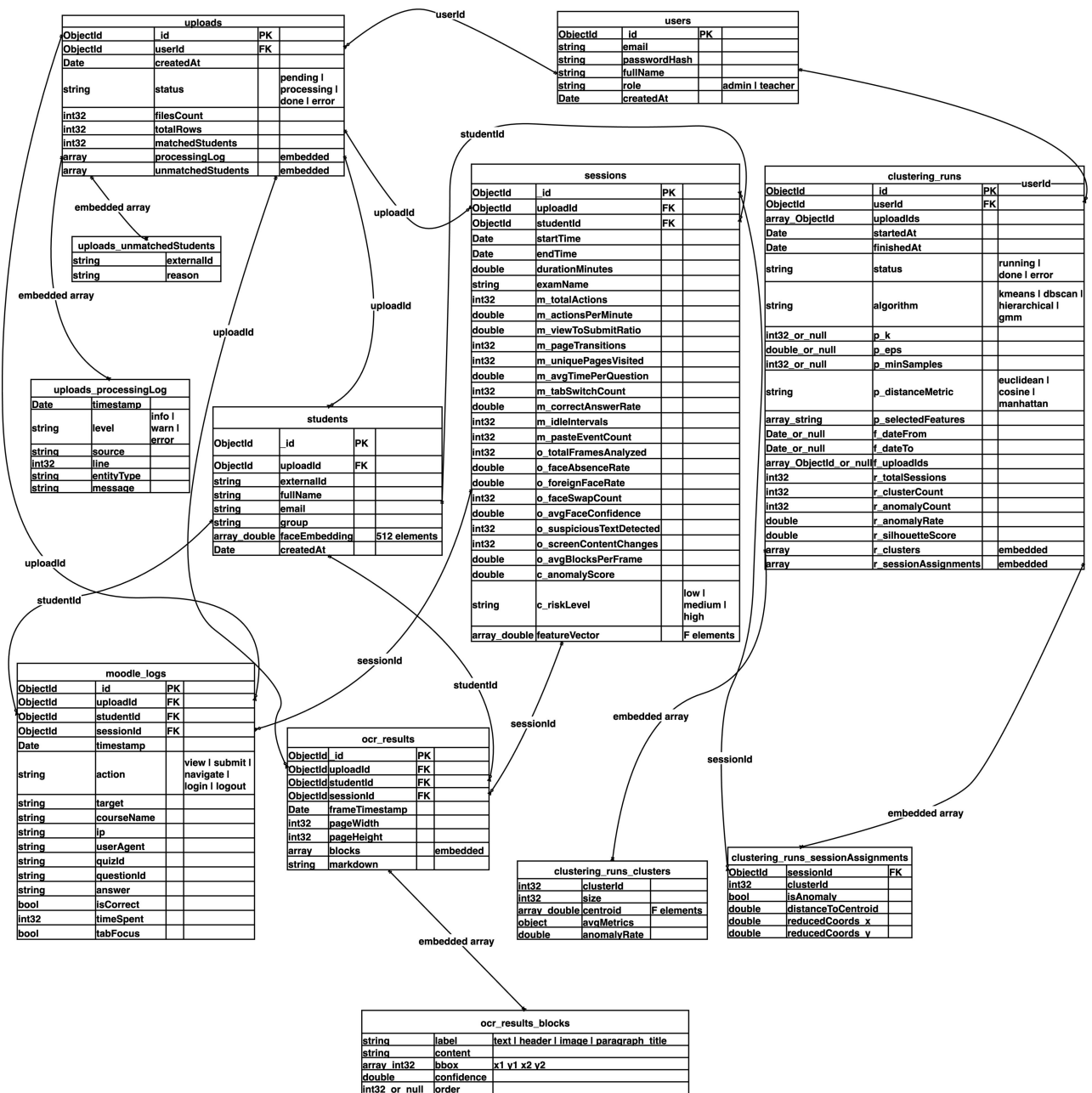
Рисунок 2 – Графическое представление NoSQL базы данных
