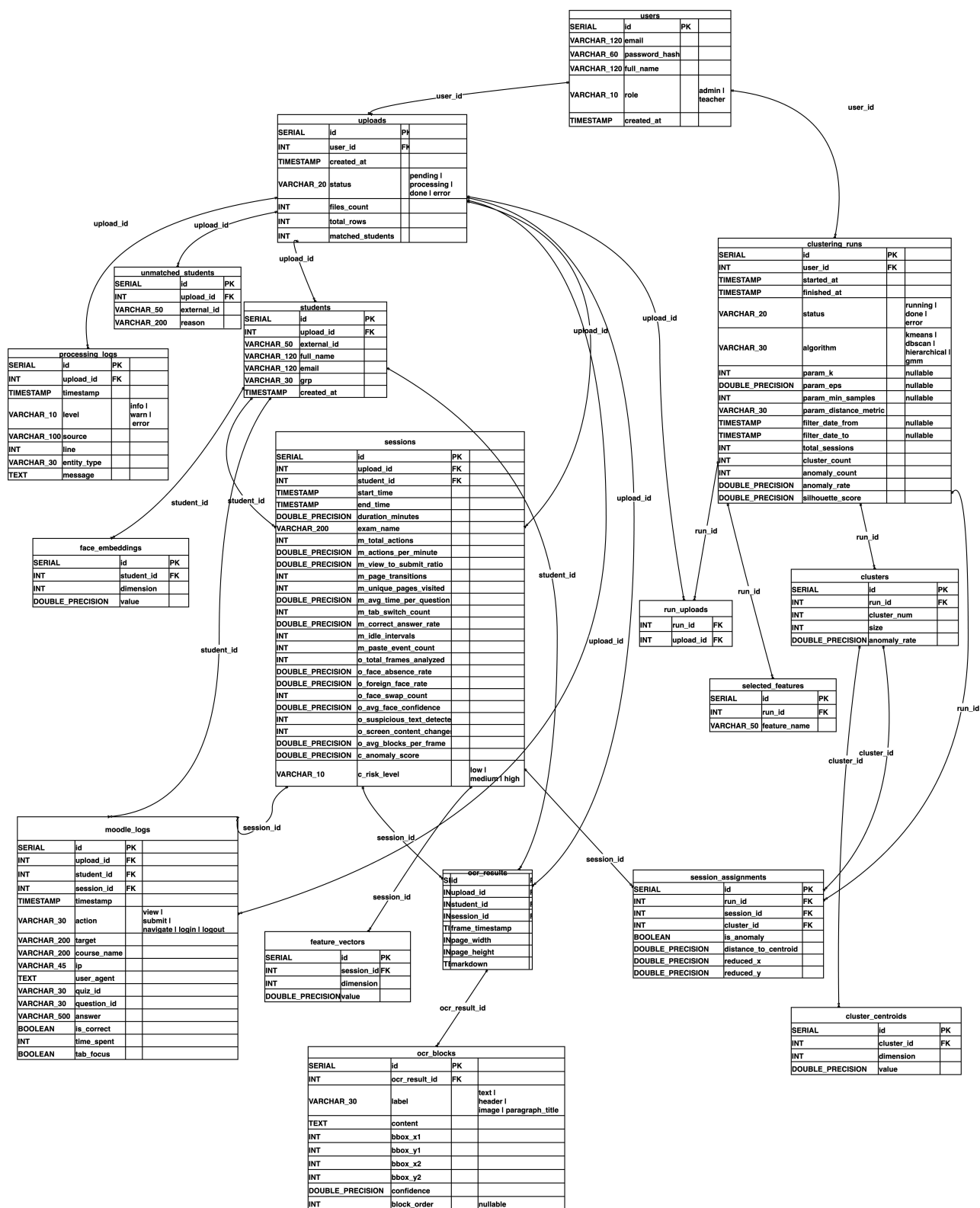
Рисунок 3 – Графическое представление SQL базы данных
