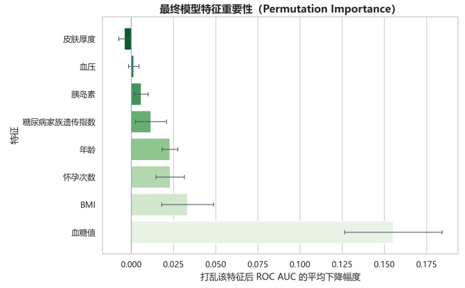
图 8. 最终模型特征重要性 (Permutation Importance)
