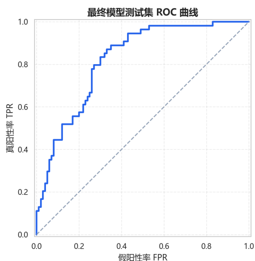
(b) ROC 曲线
