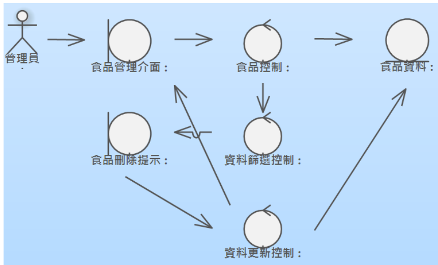
圖 24：使用案例 8.3 刪除食品強韌圖
