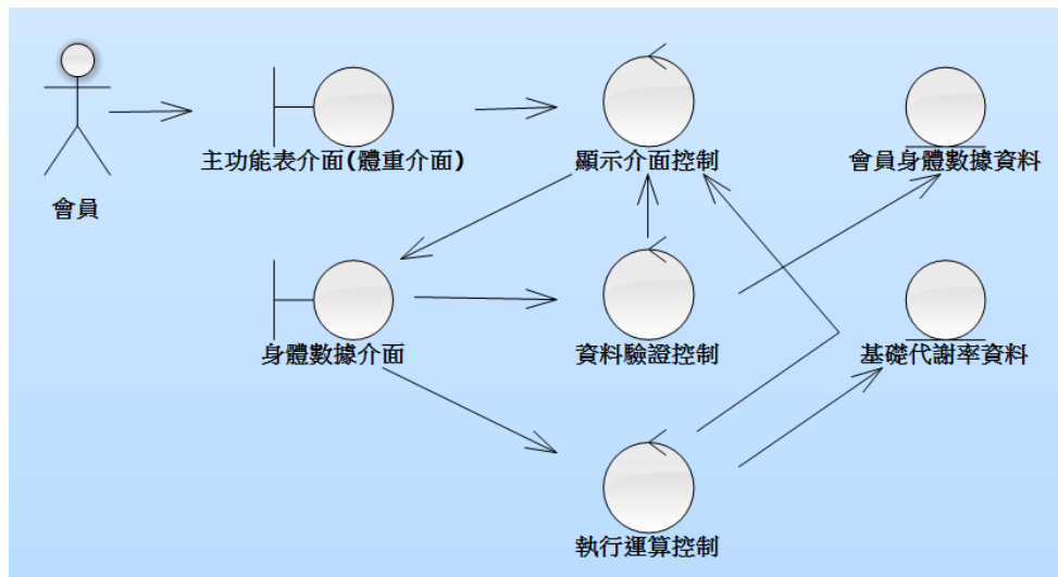
圖 10：使用案例 2.1 輸入基本數值強韌圖
