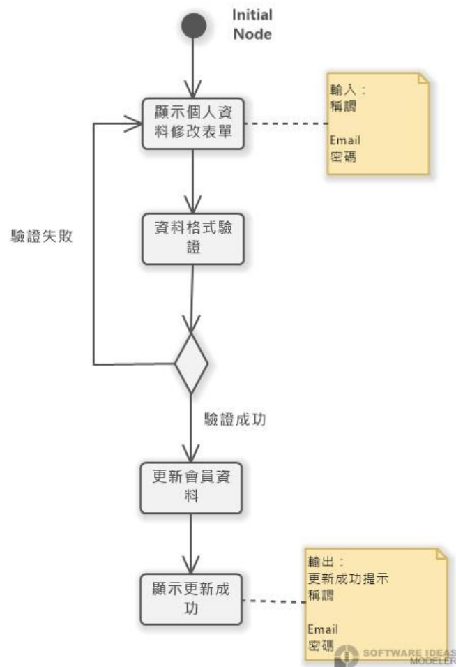
圖 5：使用案例 1.3 會員修改基本資料活動圖
