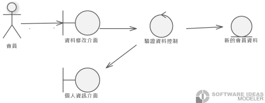
圖 6：使用案例 1.3 會員修改基本資料強韌圖
