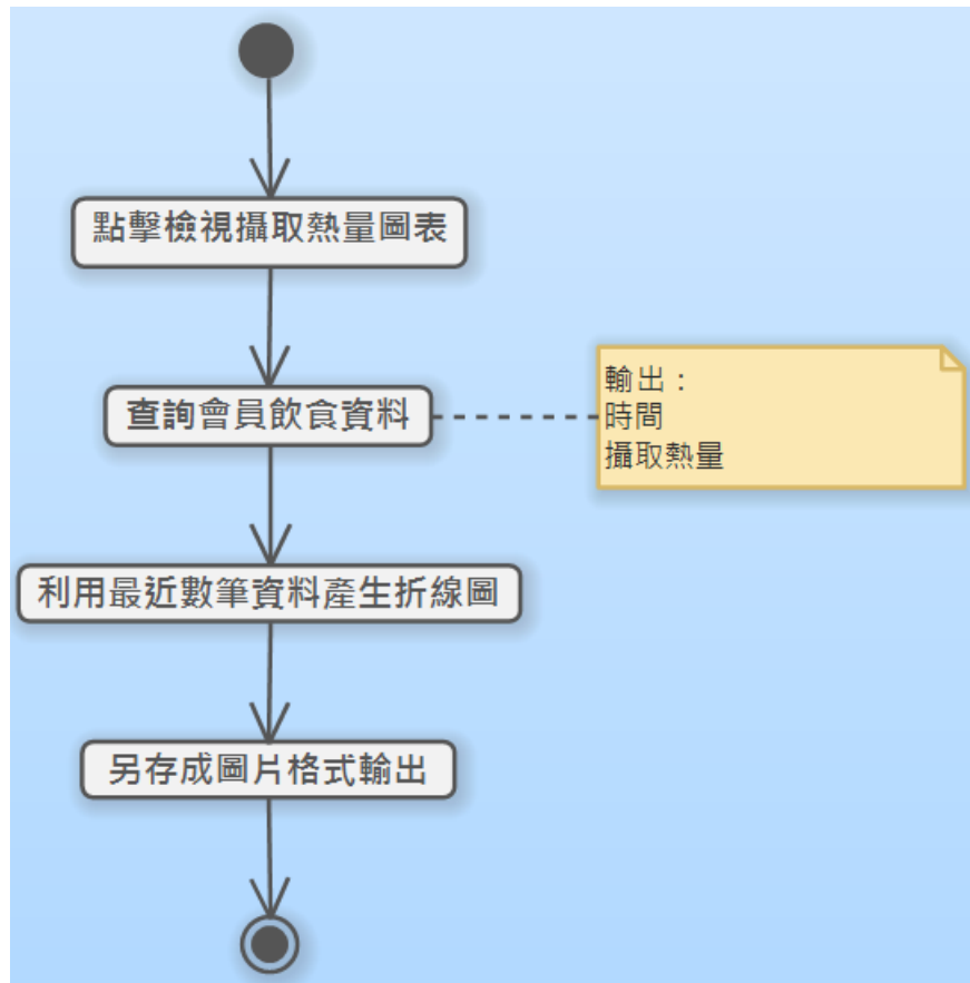
圖 17：使用案例 7.2 檢視攝取熱量圖表活動圖
