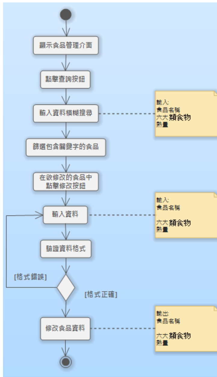
圖 21：使用案例 8.2 修改食品活動圖
