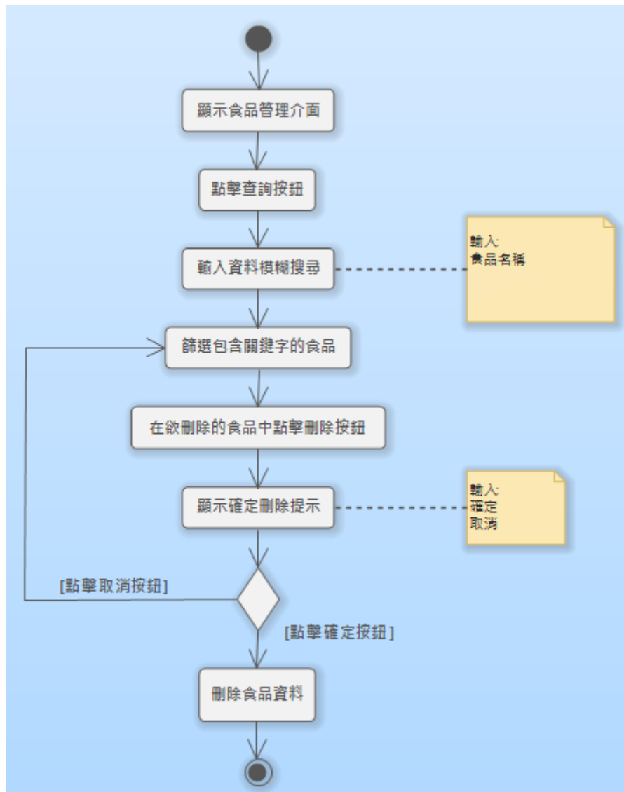
圖 23：使用案例 8.3 刪除食品活動圖
