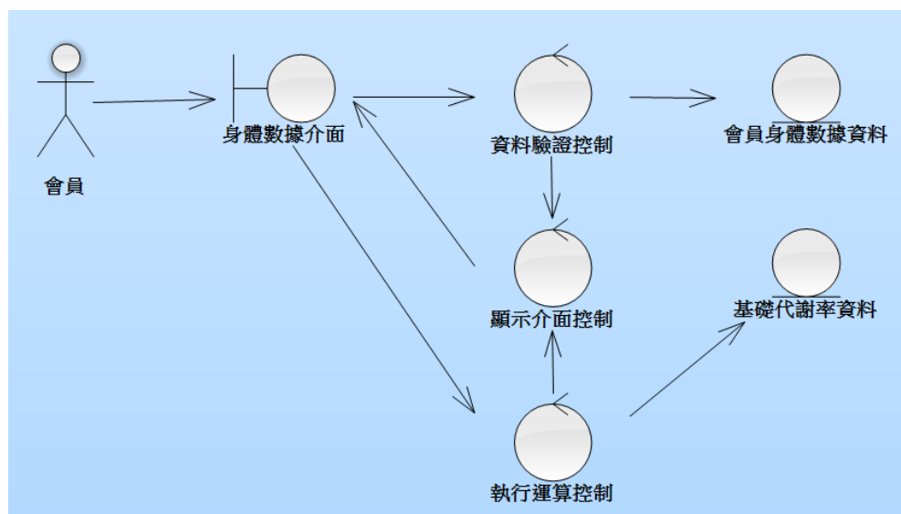
圖 12：使用案例 2.2 修改基本數值強韌圖
