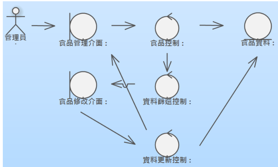
圖 22：使用案例 8.2 修改食品強韌圖
