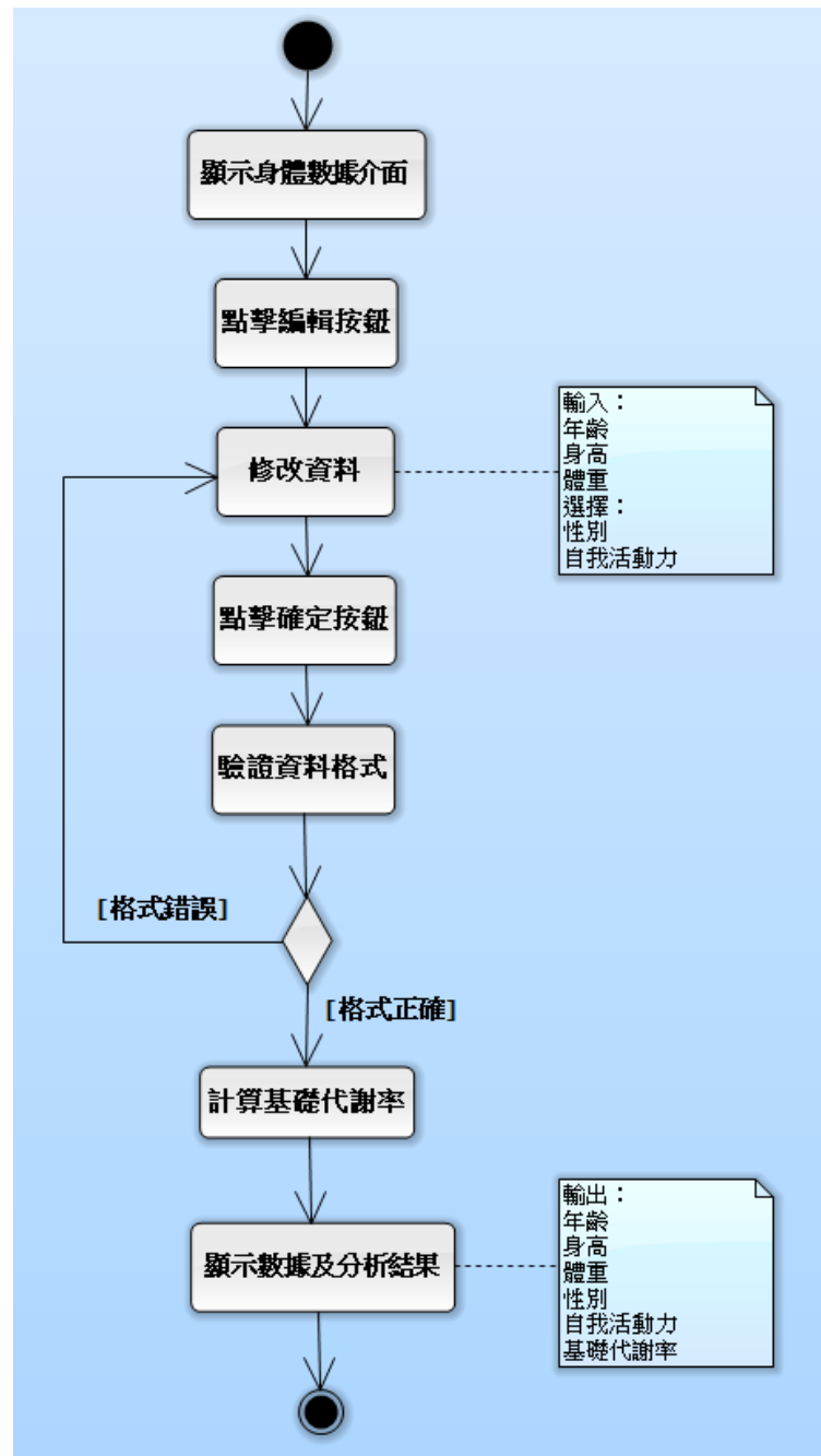
圖 11：使用案例 2.2 修改基本數值活動圖
