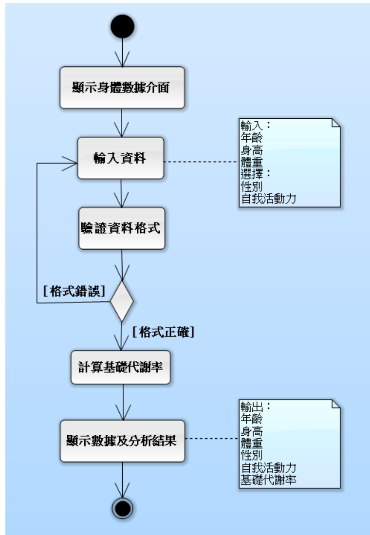
圖 9：使用案例 2.1 輸入基本數值活動圖
