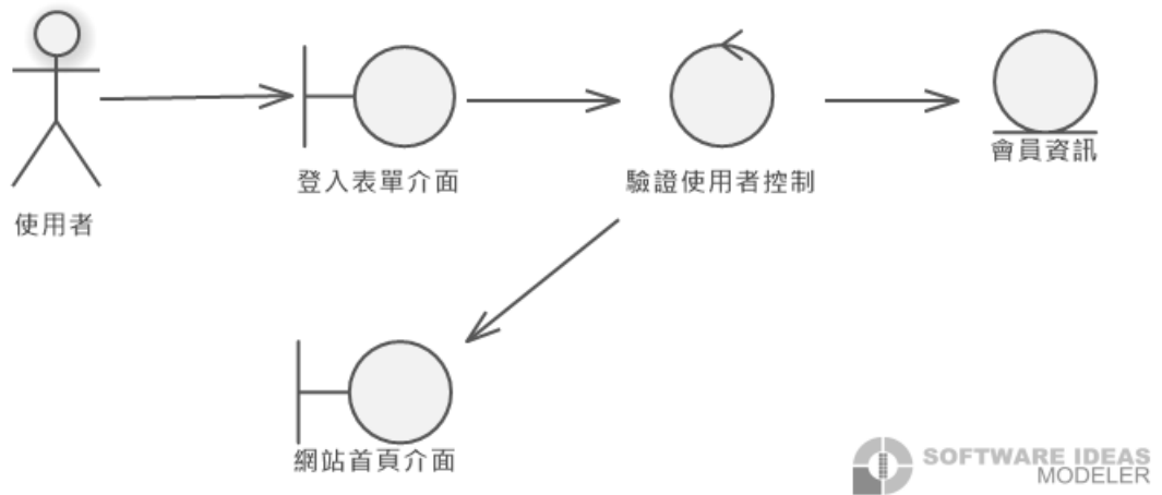
圖 4：使用案例 1.2 帳號登入強韌圖
