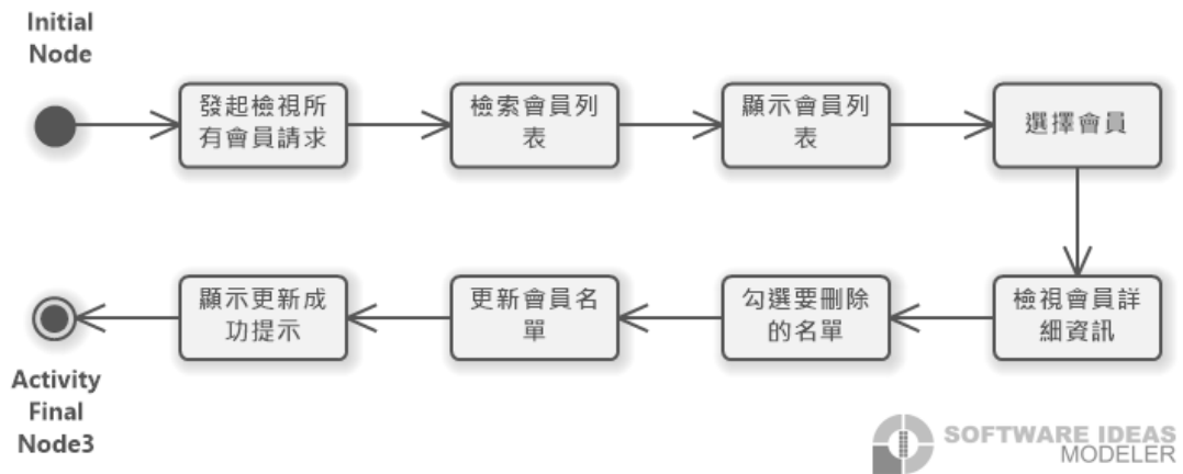
圖 7：使用案例 1.4 刪除會員活動圖
