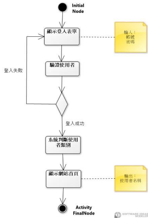
圖 3：使用案例 1.2 帳號登入活動圖
