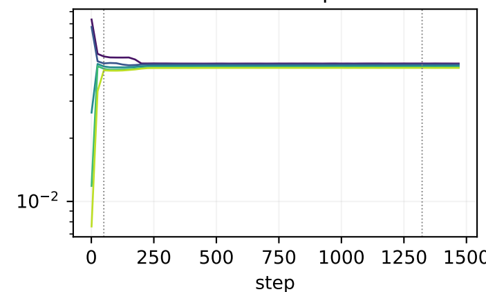
block08.down
