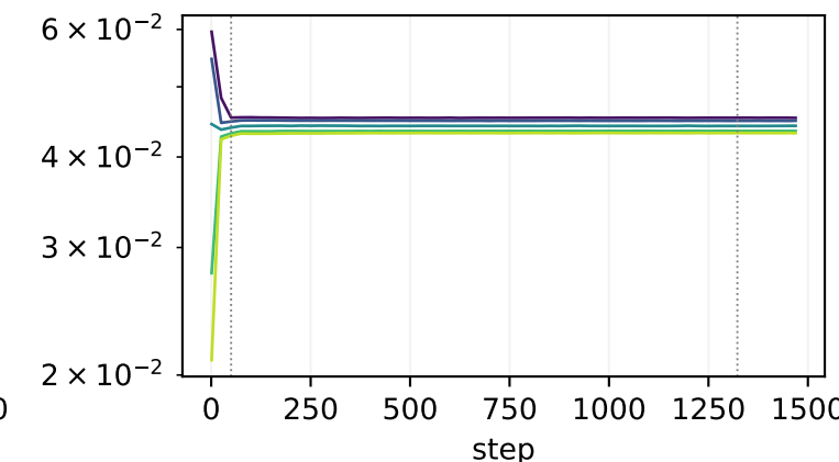
block08.down
