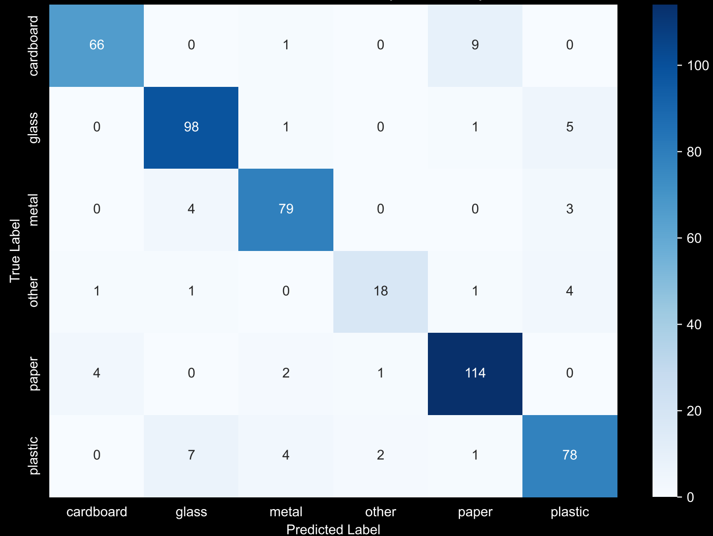
RQ1 – Confusion Matrix (ResNet-50)
